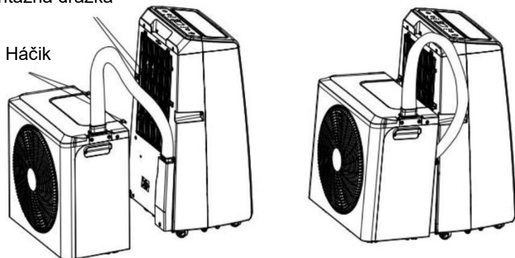
Montážna drážka
