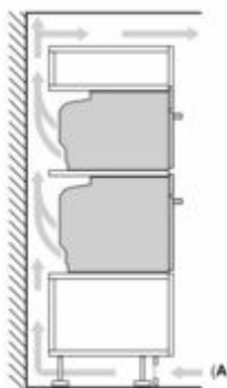
A: Air inlet \geq 200 cm 2
