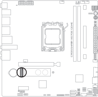
M.2(SOCKET3)
