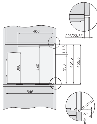
Seitenansicht H7000 M, Skizze, GB, AU
