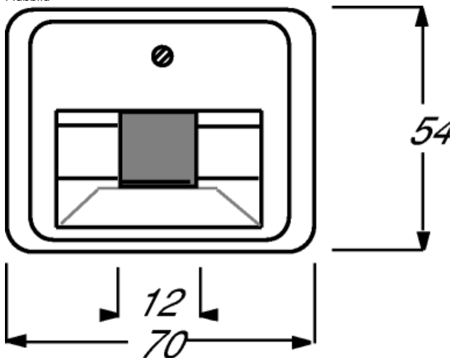
Maßbild
