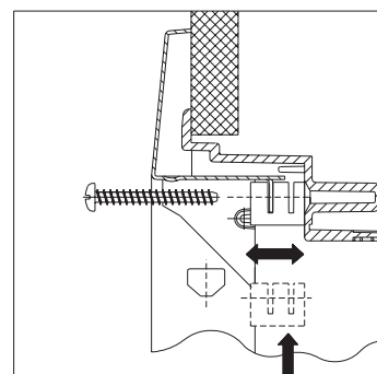
7. Maximaler Putzausgleich durch Einschieben des Distanzteils in verschiedenen Höhenstellungen.
