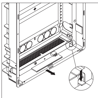
1. Schieber entnehmen (Rastungen li/re betätigen).
