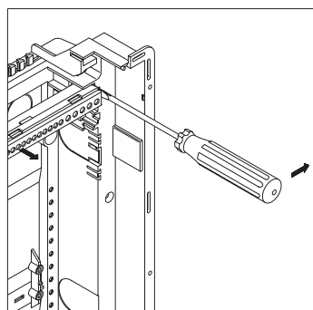
5. Zum Einbau die PE/N-Klemme einrasten, zum Ausbau Werkzeug verwenden.
