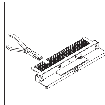
4. Schieber entsprechend den Leitungen ausbrechen.
