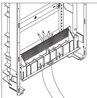
2. Leitungen einlegen. 3. Schieber parken bis Leitungsverlegung abgeschlossen.
