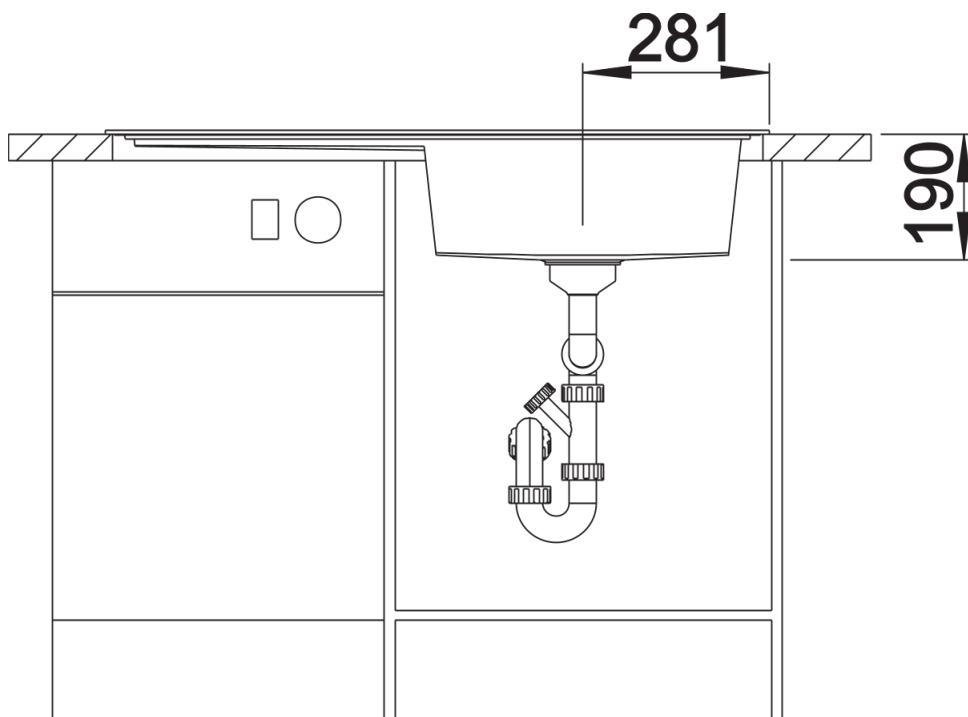
Frontansicht
