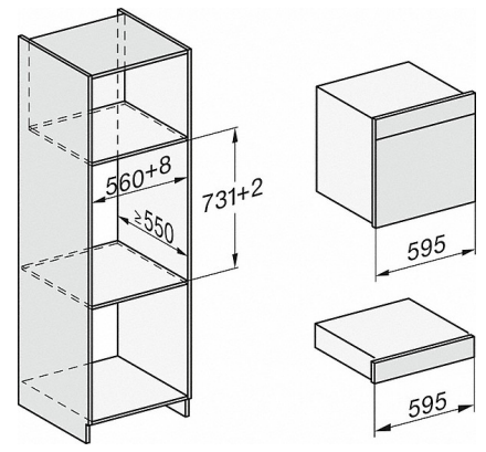
ESW7x10, EVS 7010 Skizze
