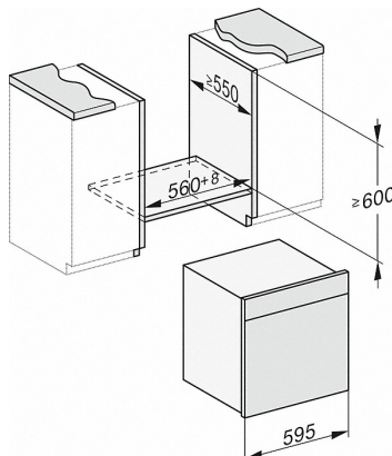
DGC7x6x, DGC7x6xX Skizze
