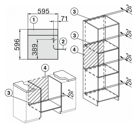
DGC7x60, DGC7x60X Skizze
