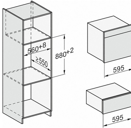
ESW7x20, Skizze
