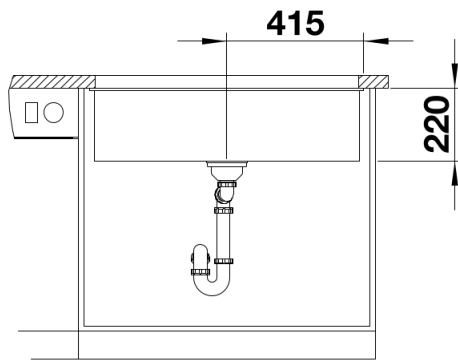
Frontansicht
