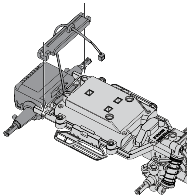
Druckplatte / Pressure Strip A7 1x
