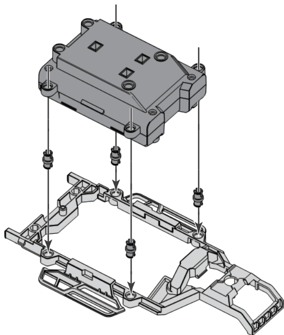
Verbinder / Latch C1 4x
