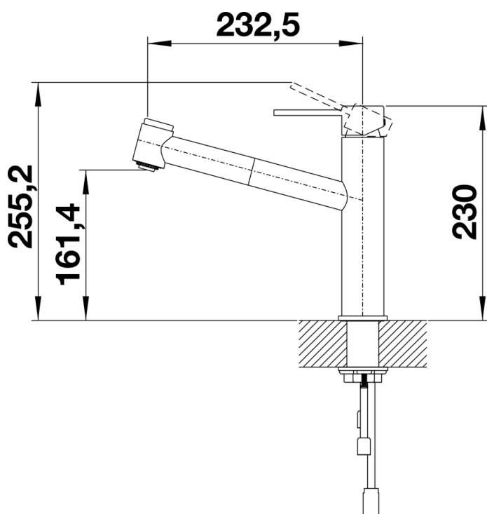
Seitenansicht
