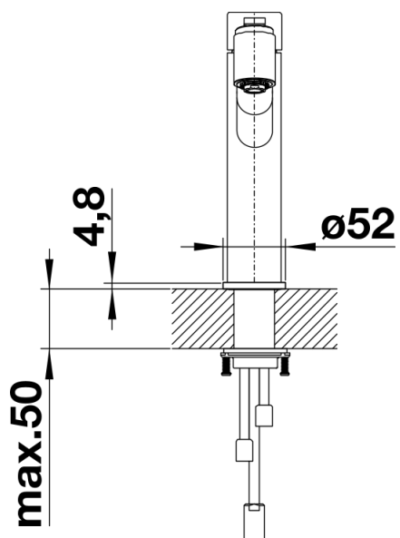
Seitenansicht Hebel 2D
