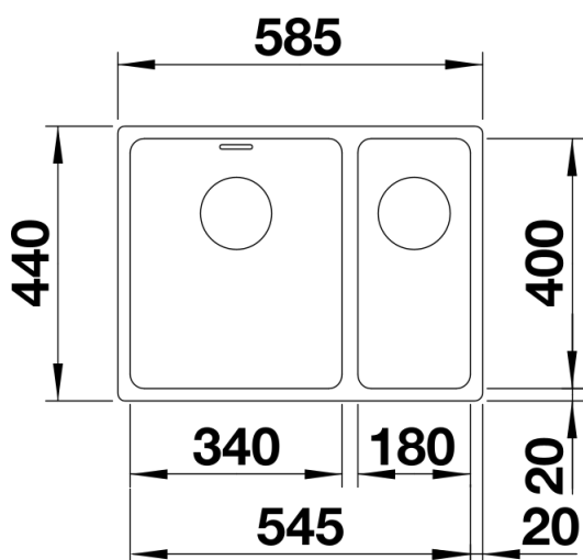
Aufsicht
