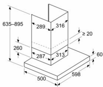
Maße in mm Gerät im Abluftbetrieb
