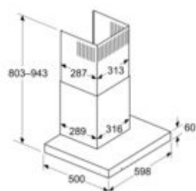
Maße in mm Ansicht Umluft
