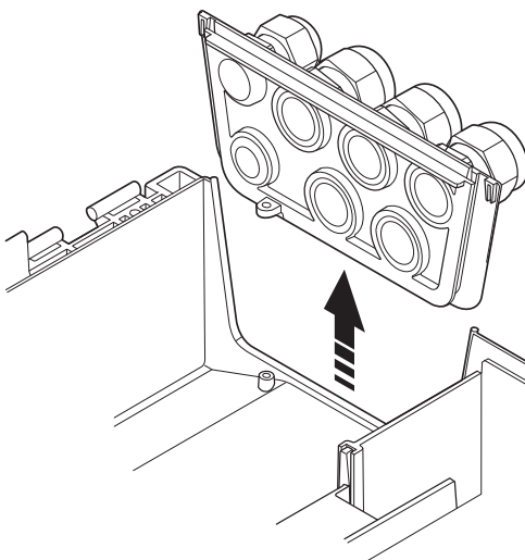
Bild 5 Flanschplatte
