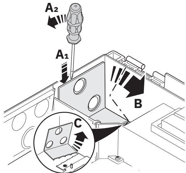
Bild 6 Schirmblech
