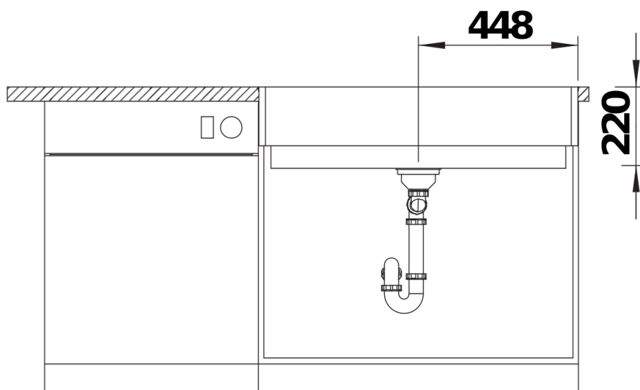
Frontansicht
