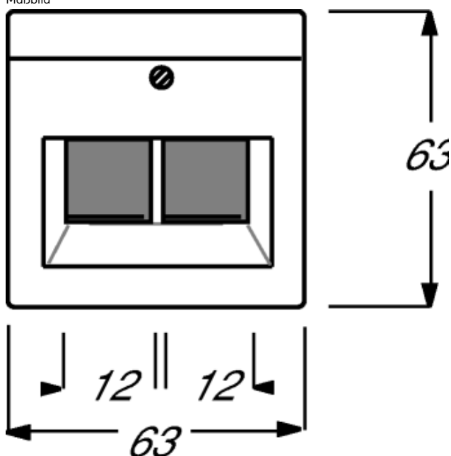
Maßbild
