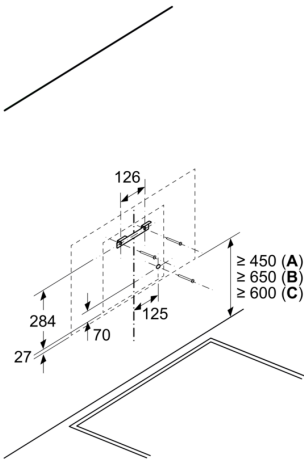
Maße in mm Wandinstallation ohne Kamin
