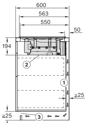
1) vorn, 2) abnehmbare Auffangwanne, 3) Reinigungsklappe, 4) Netzanschlusskasten mit Netzanschlussleitung, L = 1600 mm, 5) Dicke der Arbeitsplatte, Ablauf- und geführter Umluftbetrieb: \geq 10 mm, Pluq&Play-Betrieb: \geq 10 mm \leq 40 mm.
