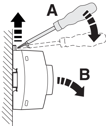
Bild 13 Abheben der Stromversorgung von der Tragschiene
