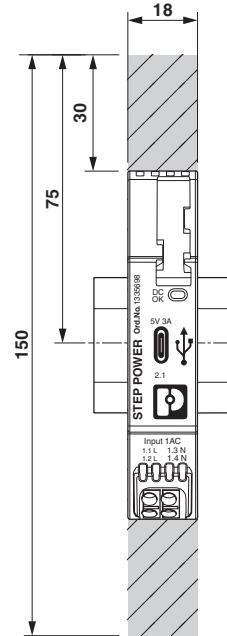
Bild 9 Geräteabmessungen und minimale Sperrflächen (Maße in mm)
