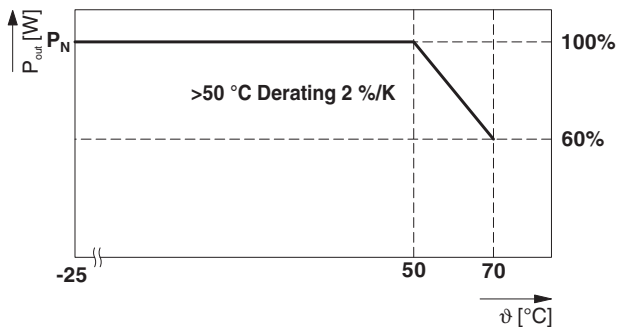
Bild 22 Ausgangsleistung in Abhängigkeit zur Umgebungstemperatur
