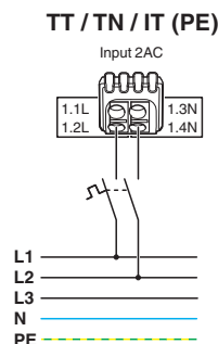
Bild 17 Prinzipdarstellung, 2-polige Absicherung
