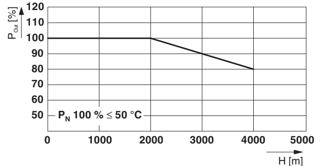
Bild 23 Ausgangsleistung in Abhängigkeit zur Aufstellhöhe
