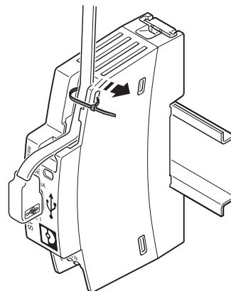
Bild 12 Zugentlastung mit Kabelbinder
