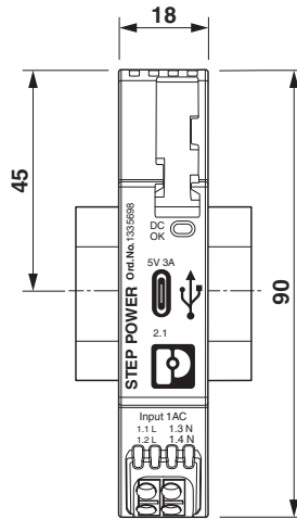
Bild 6 Geräteabmessungen (Maße in mm)
