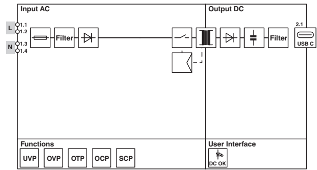
Bild 4 Blockschaltbild
