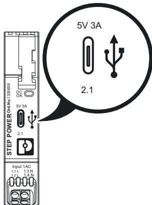
Bild 19 Lage der DC-Ausgangsbuchse
