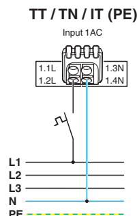
Bild 16 Prinzipdarstellung, 1-polige Absicherung
