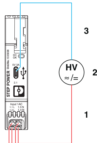
Bild 1 Potenzialbezogene Verdrahtung für den Hochspannungstest
