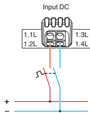
Bild 18 Prinzipdarstellung, 2-polige Absicherung
