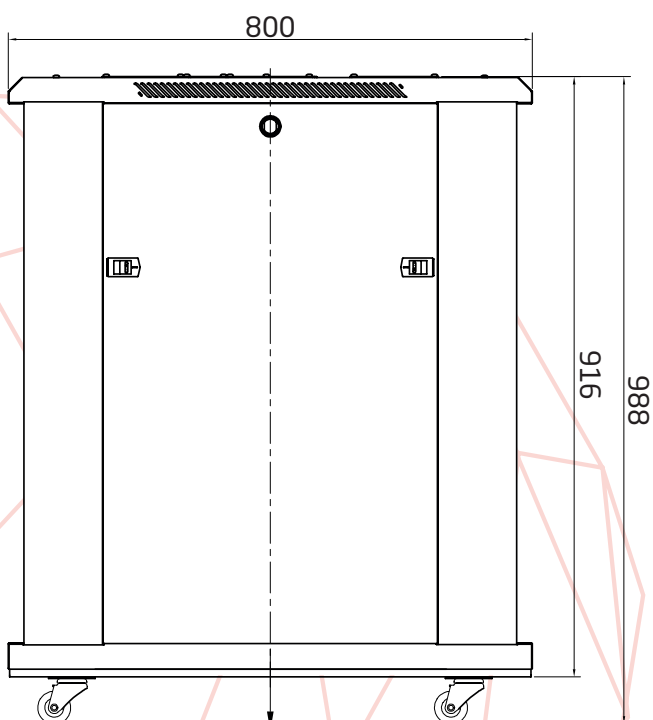
Seitenansicht
