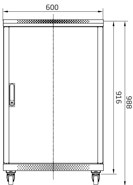
Hinteransicht
