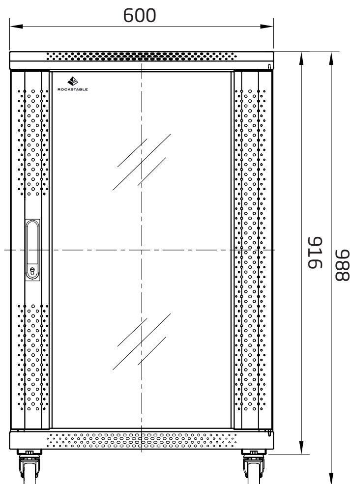
Vorderansicht
