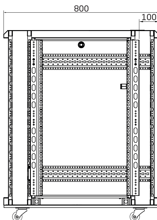
Seiteninnenansicht
