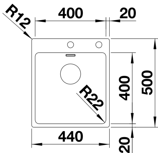
Aufsicht
