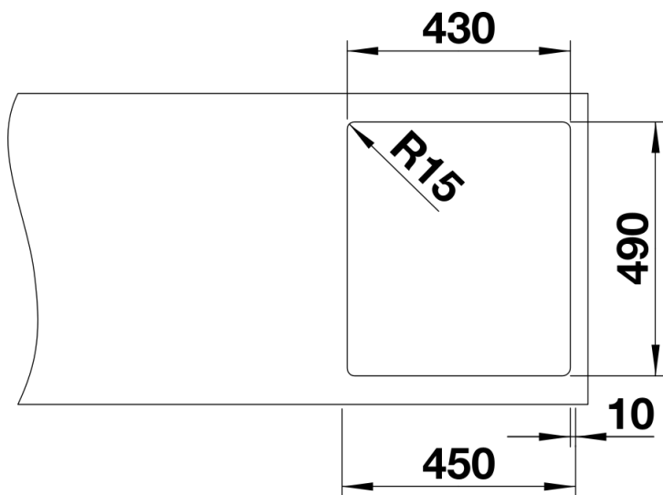
Ausschnitt
