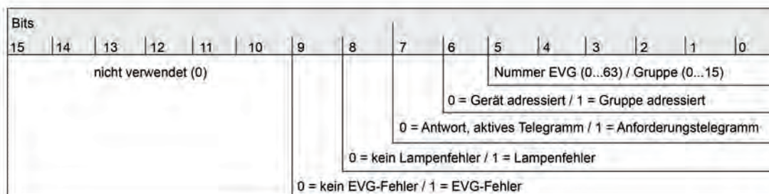
Bild 27: Telegrammaufbau 2-Byte KNX-Fehlerstatus
