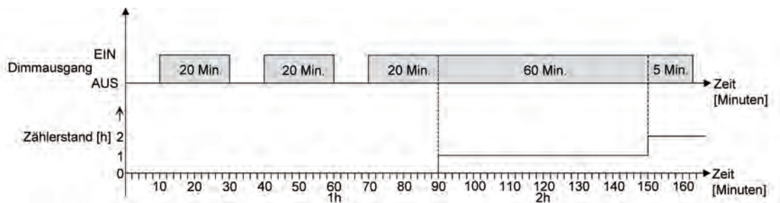
Bild 52: Funktionsweise des Betriebsstundenzählers (am Beispiel eines Vorwärtzählers)
