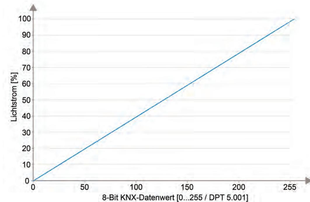
Bild 33: Lineare DALI-Dimmkennlinie (relativer Lichtstrom [%] abhängig vom 8-Bit KNX Datenwert [0...255])
