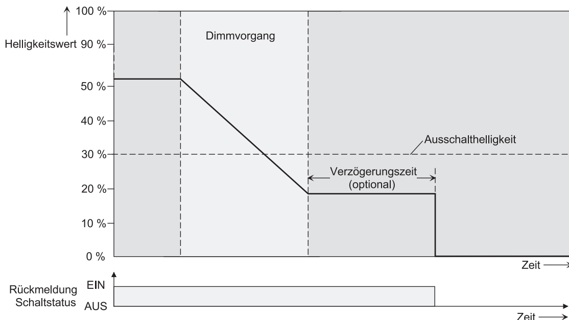
Bild 41: Dimm- und Schaltverhalten der automatischen Ausschaltfunktion
