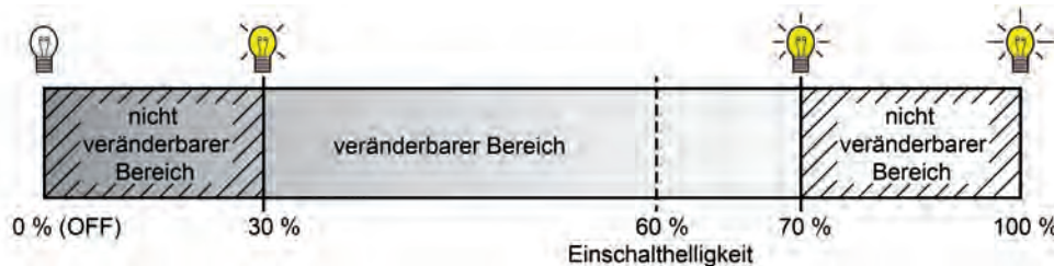
Bild 30: Beispiel eines Helligkeitsbereichs mit Einschalthelligkeit
