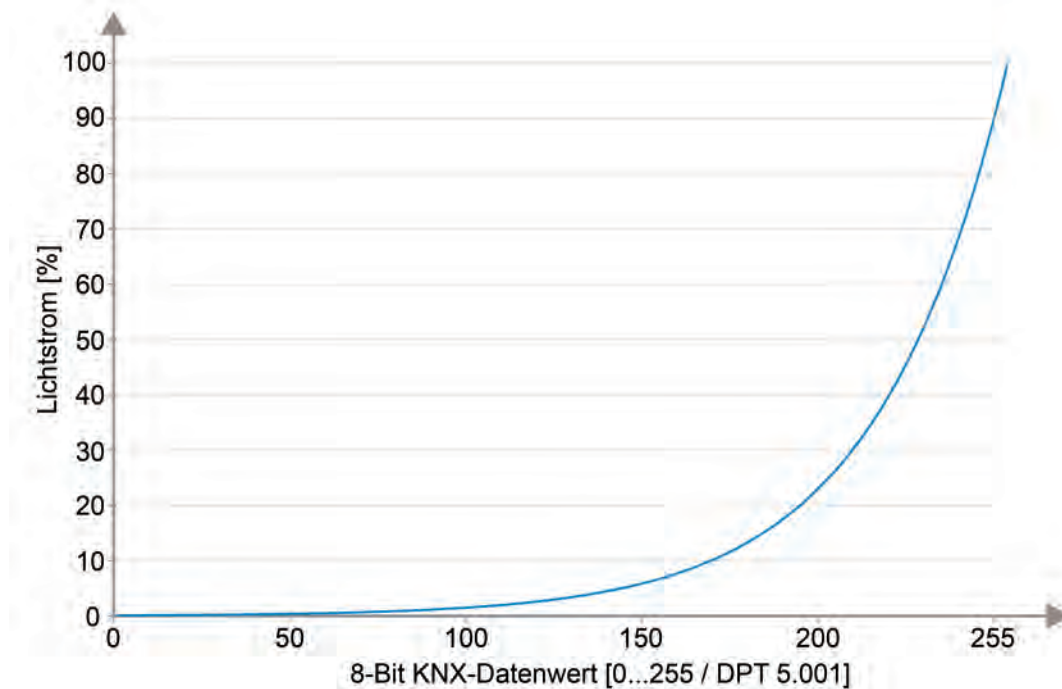
Bild 34: Logarithmische DALI-Dimmkennlinie (relativer Lichtstrom [%] abhängig vom 8-Bit KNX Datenwert [0...255])
