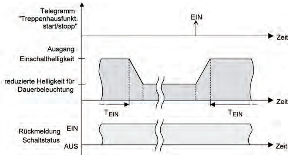
Bild 50: Die Dauerbeleuchtung der Treppenhausfunktion mit Soft-AUS-Funktion
