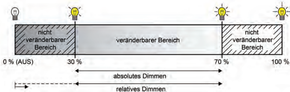
Bild 31: Beispiel eines dimmbaren Helligkeitsbereichs
