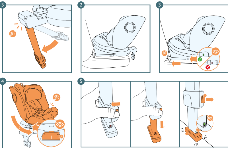
A: Stabilisierungsfuß
