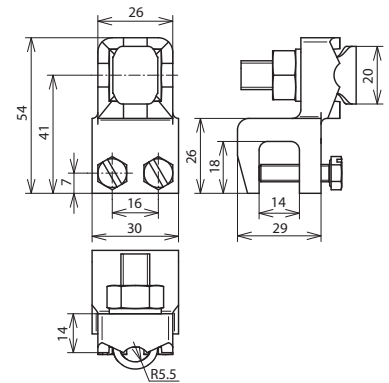
Maßbild
