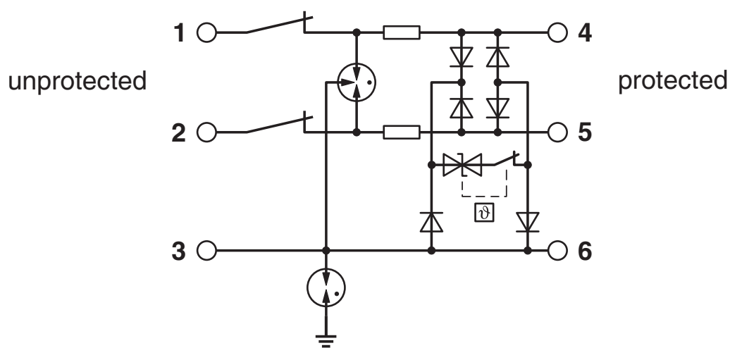
Schaltplan
