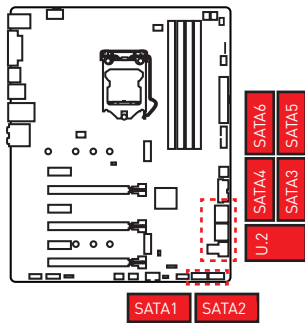
1xU.2+ 6xSATA
