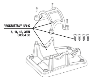
JBL ProCristal UV-C 5,11,18,36 W Halterung
