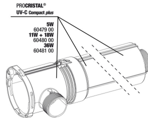
JBL ProCristal UV-C Compact plus Gehäuse Set
