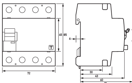
Maßzeichnung Fehlerstromschutzschalter DFS 4 063-4/0,10-A
