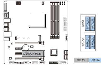
1x M.2 SATA SSD Slot -- 5x SATA HDDs
