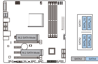
2x M.2 SATA SSD Slot -- 5x SATA HDDs
