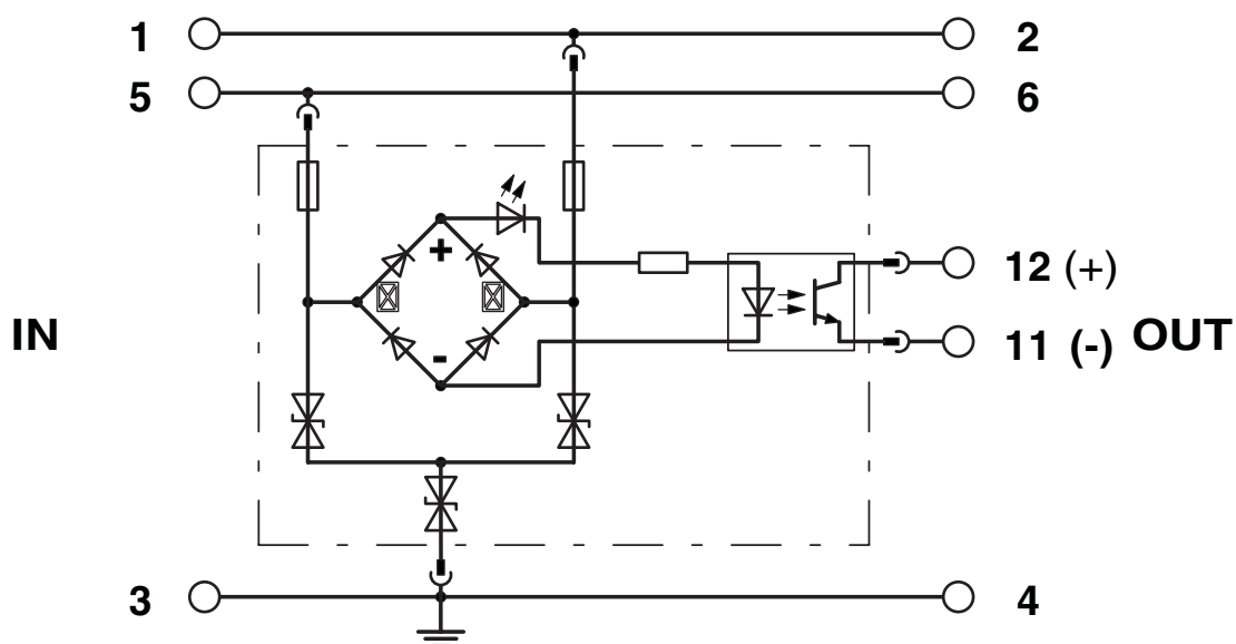
Schaltplan
