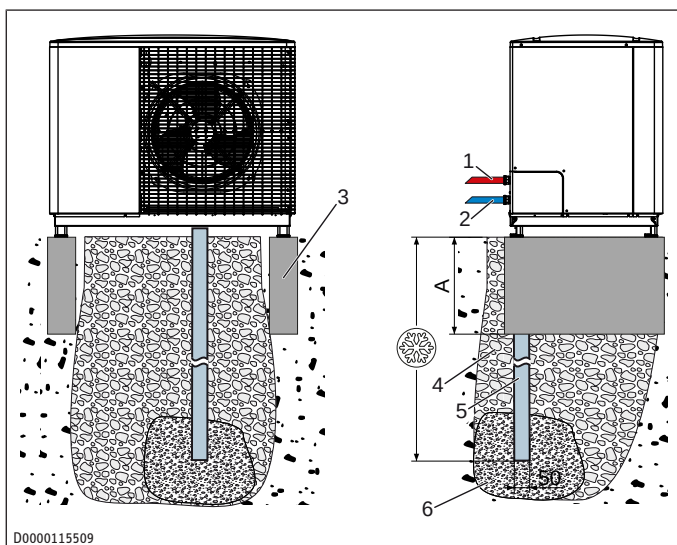
1 Heizung Vorlauf 2 Heizung Rücklauf 3 Streifenfundament (Kantenstein) 4 Schotter 5 Kondensatablaufrohr 6 Kiesbett
