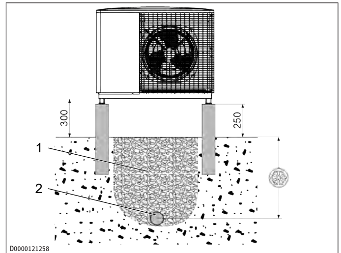
1 Schotter 2 Drainagerohr
