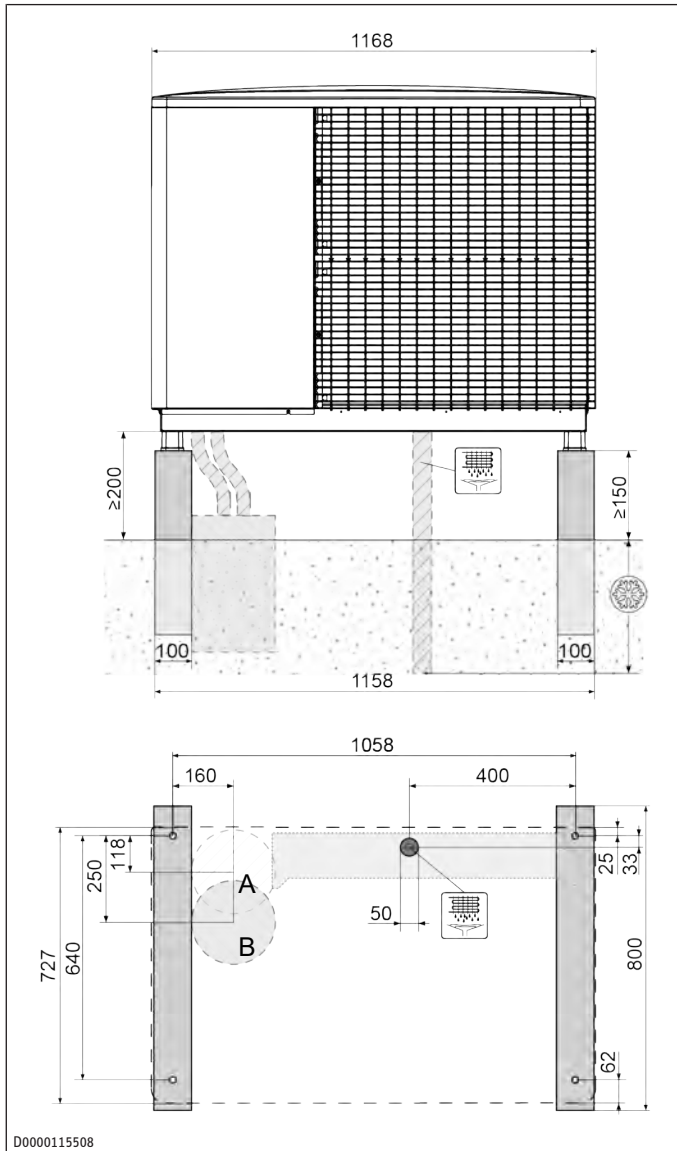
A Hydraulische Anschlüsse mit Kondensatwanne B Hydraulische Anschlüsse ohne Kondensatwanne
