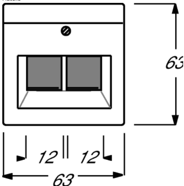
Maßbild
