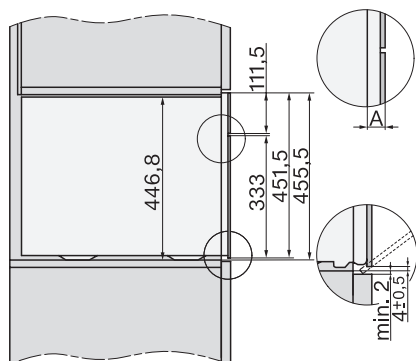
DGC7x4x, DGC7x4xX, DGC7x4xHCPro, DGC7x4xHCXPro Skizze
