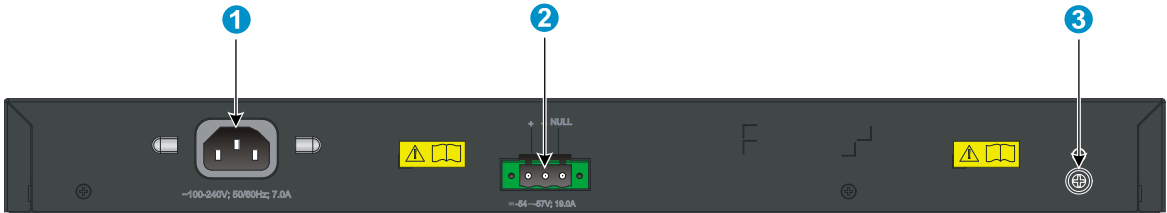
Figure 10 3600-24-PoE+ v2 EI Switch/3600-24-PoE+ v2 SI rear panel
