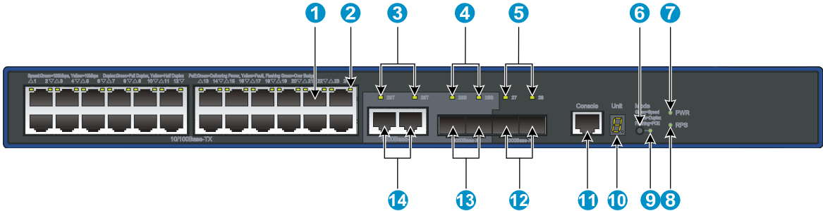
Figure 9 3600-24-PoE+ v2 EI Switch/3600-24-PoE+ v2 SI front panel
