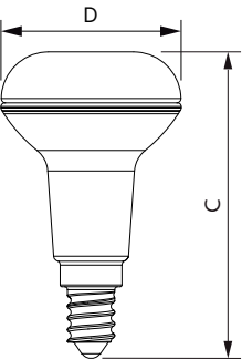
R50 4-40W 210lm 36D 2700K E14 No
