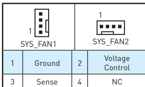
DC 模式风扇接口
