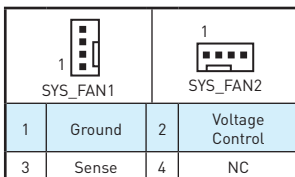
Lüfteranschluss des DC-Modus
