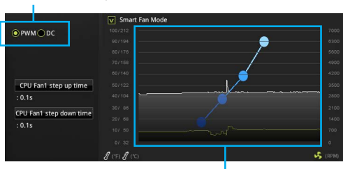
PWM 모드 또는 DC 모드 선택
