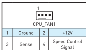
Lüfteranschluss des PWM-Modus
