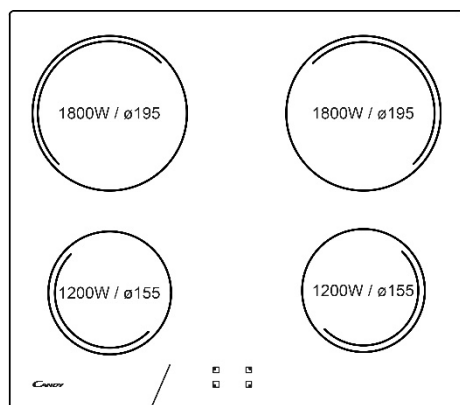
(Versione 2) Figura 3 Superficie in vetroceramica
