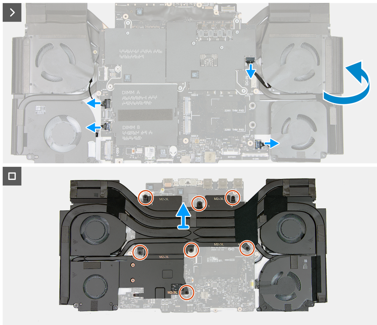
Abbildung 72. Entfernen der Lüfter- und Kühlkörperbaugruppe
