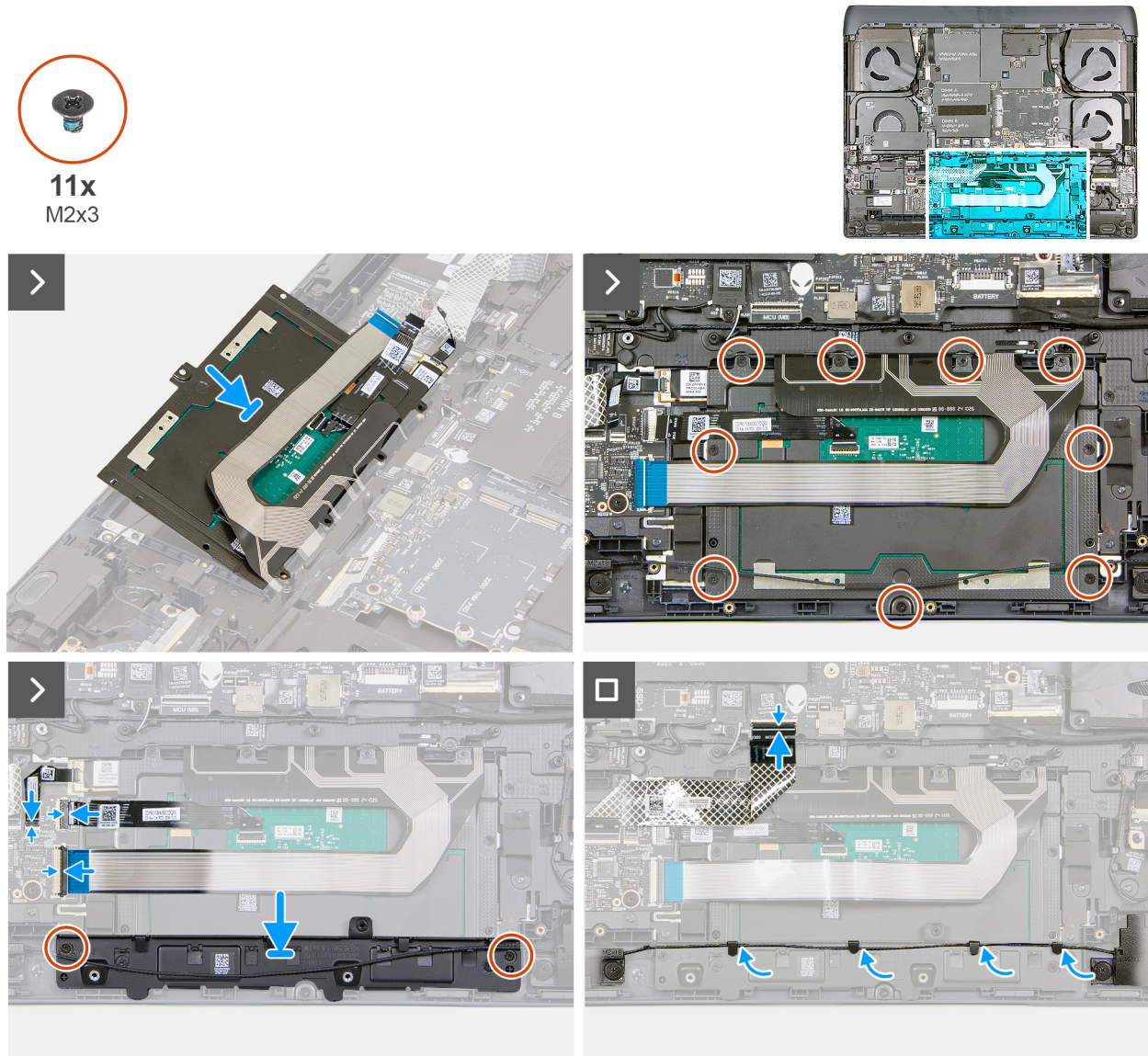
Abbildung 40. Installieren der Touchpad-Baugruppe
