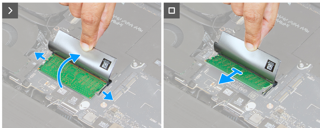
Abbildung 21. Entfernen des Arbeitsspeichermoduls
