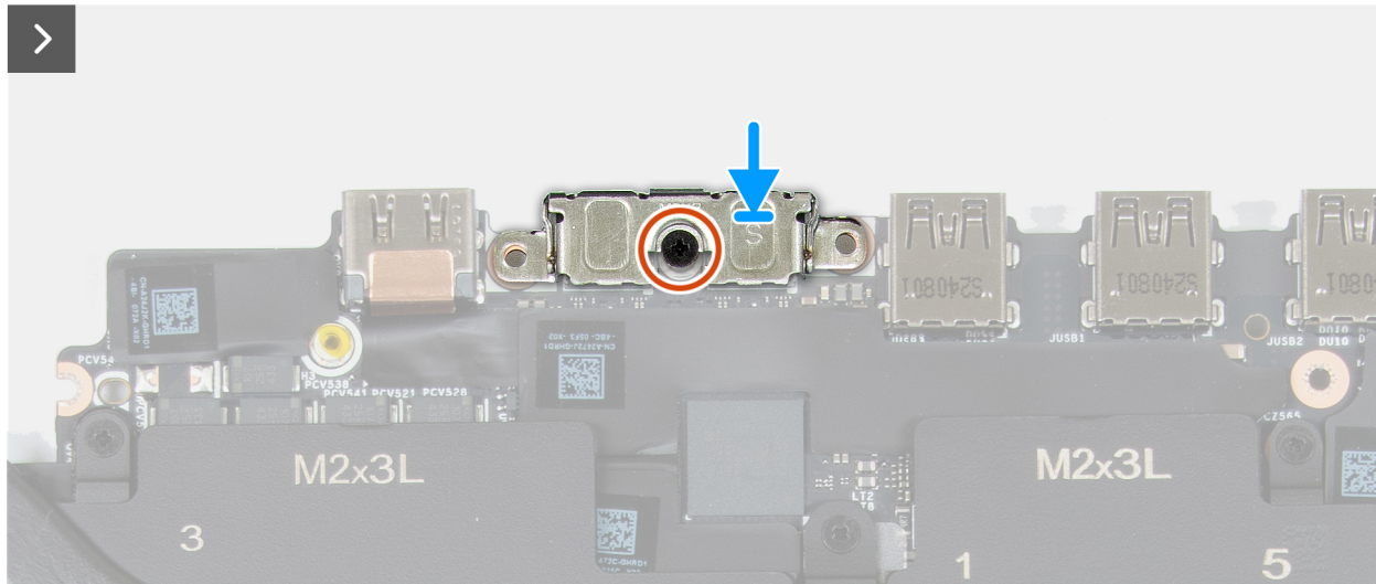
Abbildung 70. Einbauen der USB-Typ-C-Halterung
