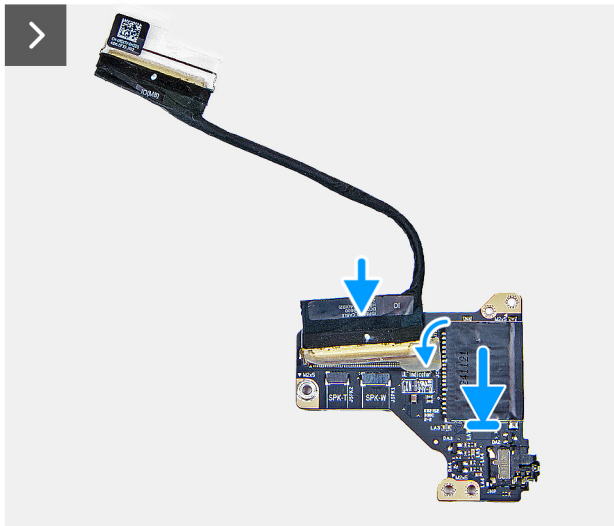
Abbildung 32. Installieren der I/O-Platine
