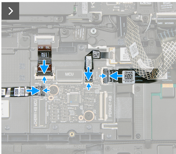
Abbildung 42. Installieren der Tastatursteuerungsplatine
