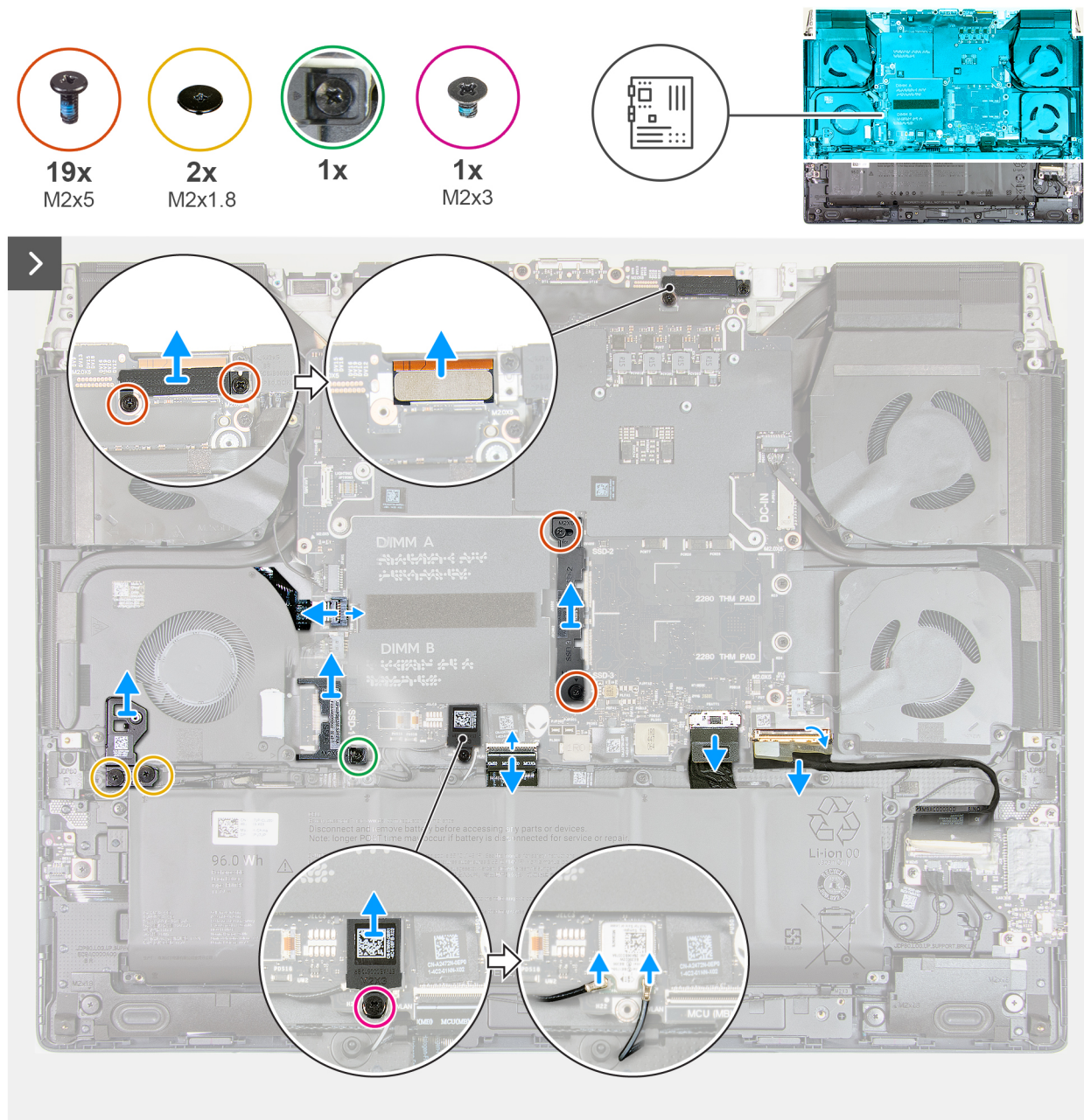
Abbildung 61. Trennen der Kabel von der Hauptplatine
