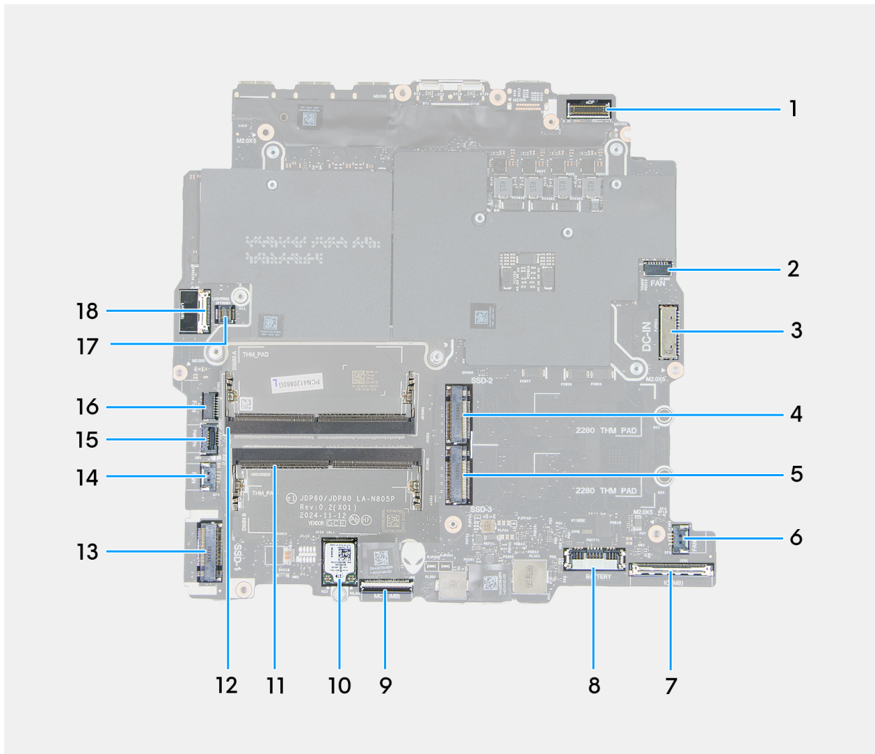
Abbildung 59. Anschlüsse auf der Hauptplatine
