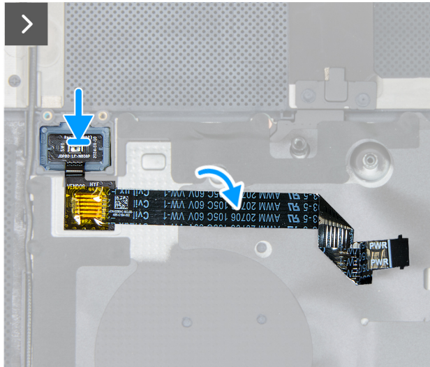
Abbildung 75. Installieren des Netzschalters
