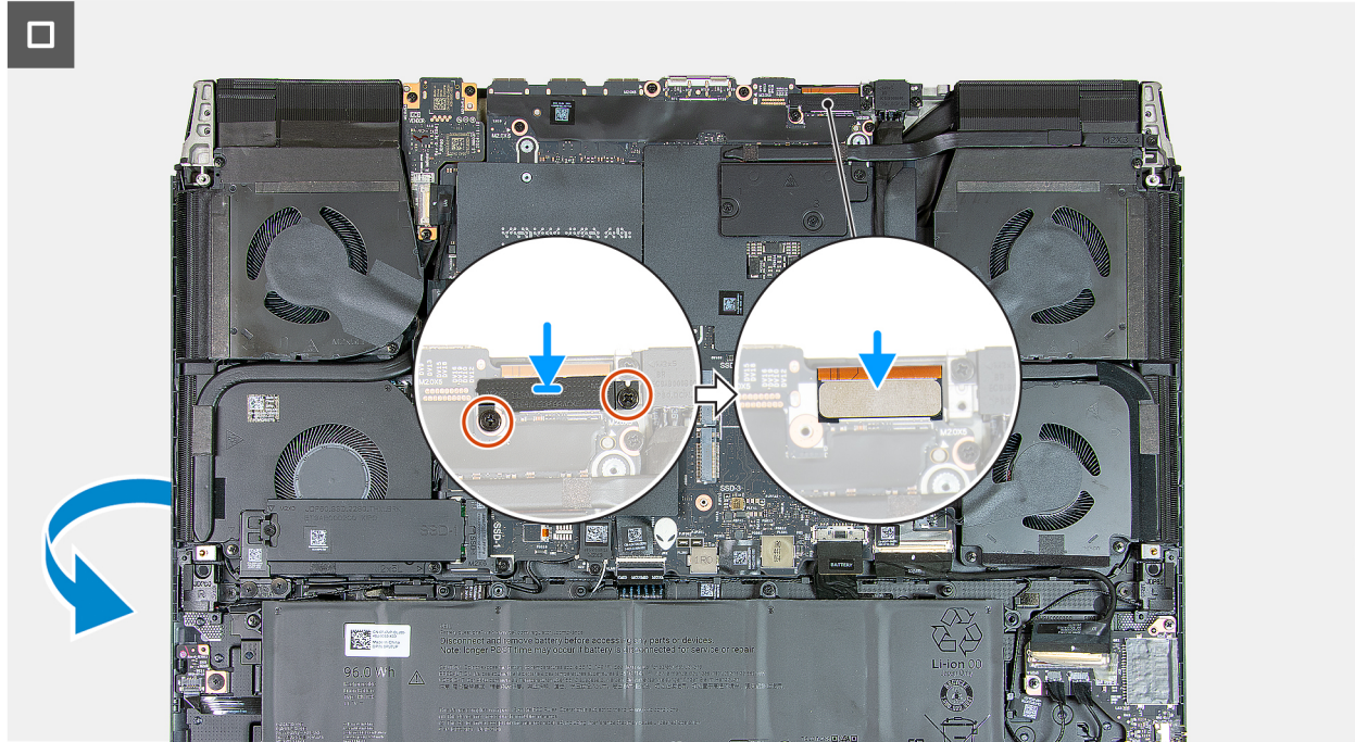
Abbildung 53. Einbauen der Displaybaugruppe
