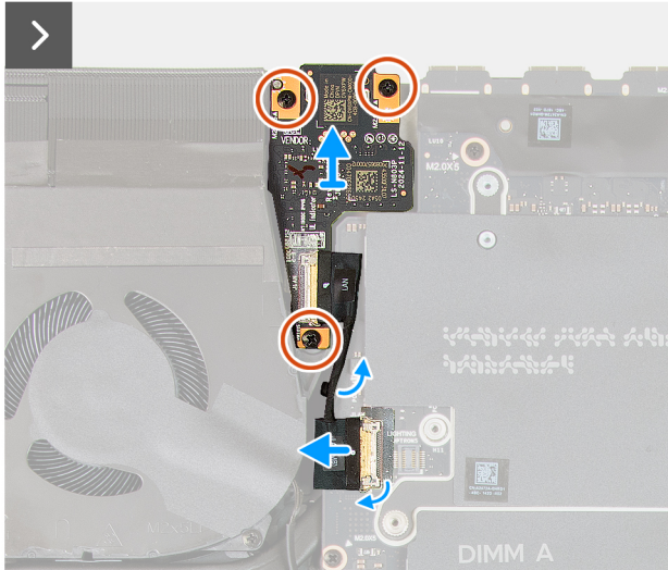
Abbildung 55. Entfernen der LAN-Platine
