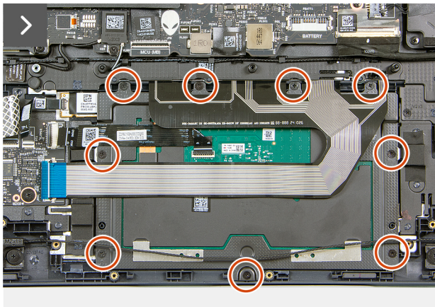
Abbildung 39. Entfernen der Touchpad-Baugruppe
