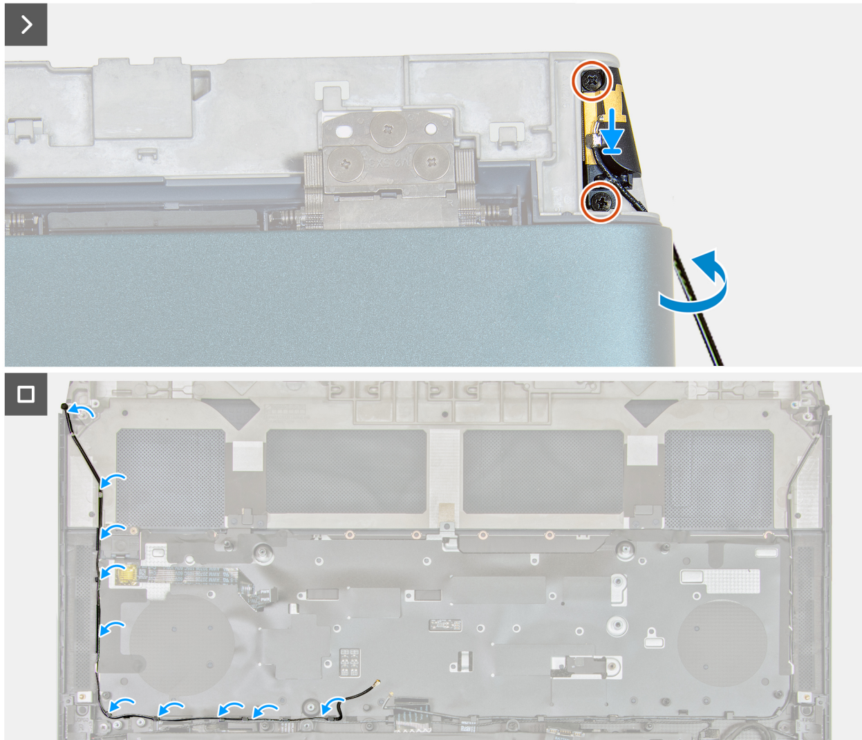
Abbildung 77. Einbauen der WLAN-Hauptantenne
