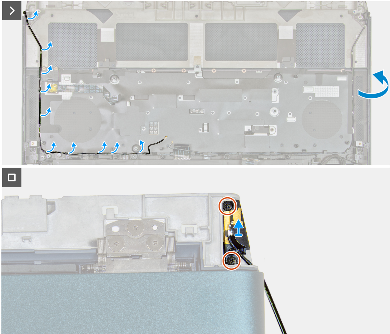
Abbildung 78. Entfernen der WLAN-Aux-Antenne
