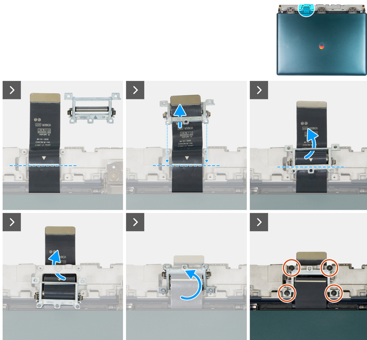
Abbildung 52. Einbauen der Displaybaugruppe
