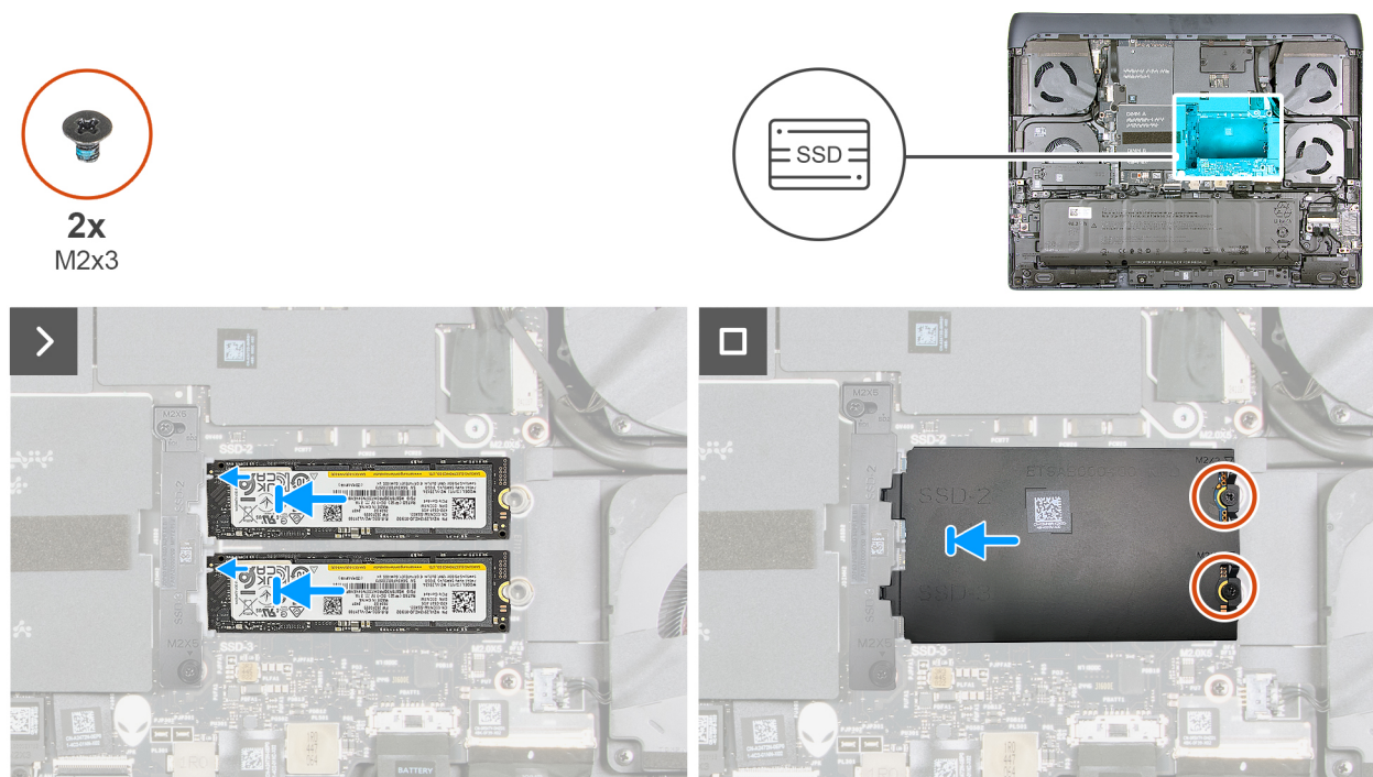
Abbildung 28. Installieren des M.2-2280-SSD in Steckplatz 2 und Steckplatz 3
