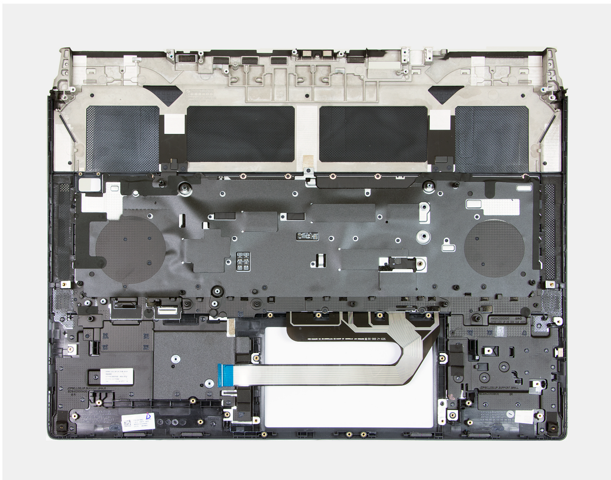
Abbildung 80. Einbauen der Handauflagen-Tastatur-Baugruppe
