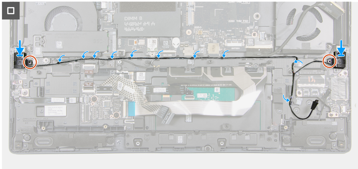
Abbildung 36. Einbauen der Hochtöner
