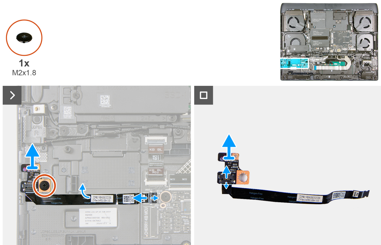
Abbildung 43. Entfernen der Hall-Sensorplatine
