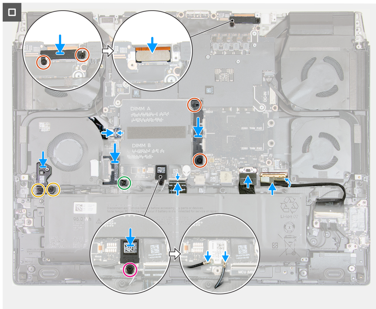
Abbildung 69. Einbauen der Systemplatine
