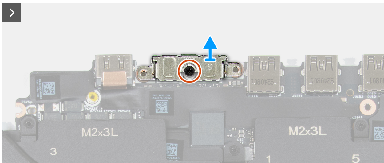
Abbildung 63. Entfernen der USB-Typ-C-Halterung
