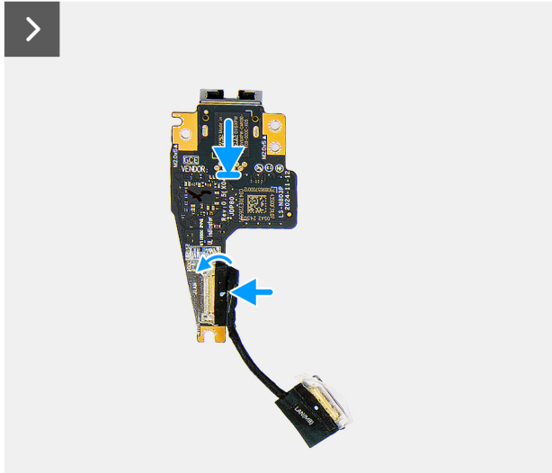
Abbildung 56. Einbauen der LAN-Platine
