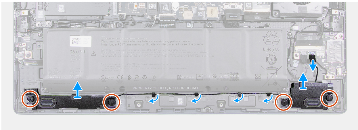
Abbildung 33. Entfernen der Woofer
