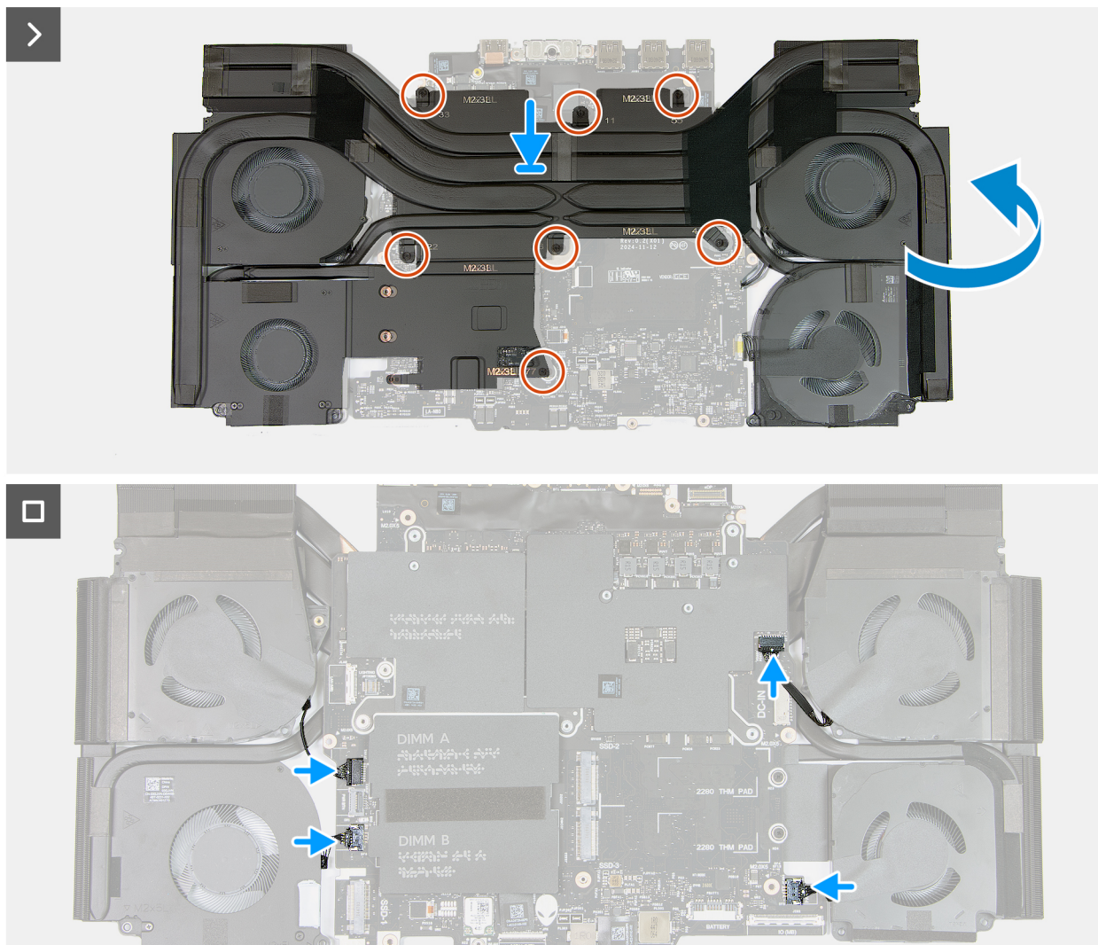
Abbildung 73. Installieren der Lüfter- und Kühlkörperbaugruppe
