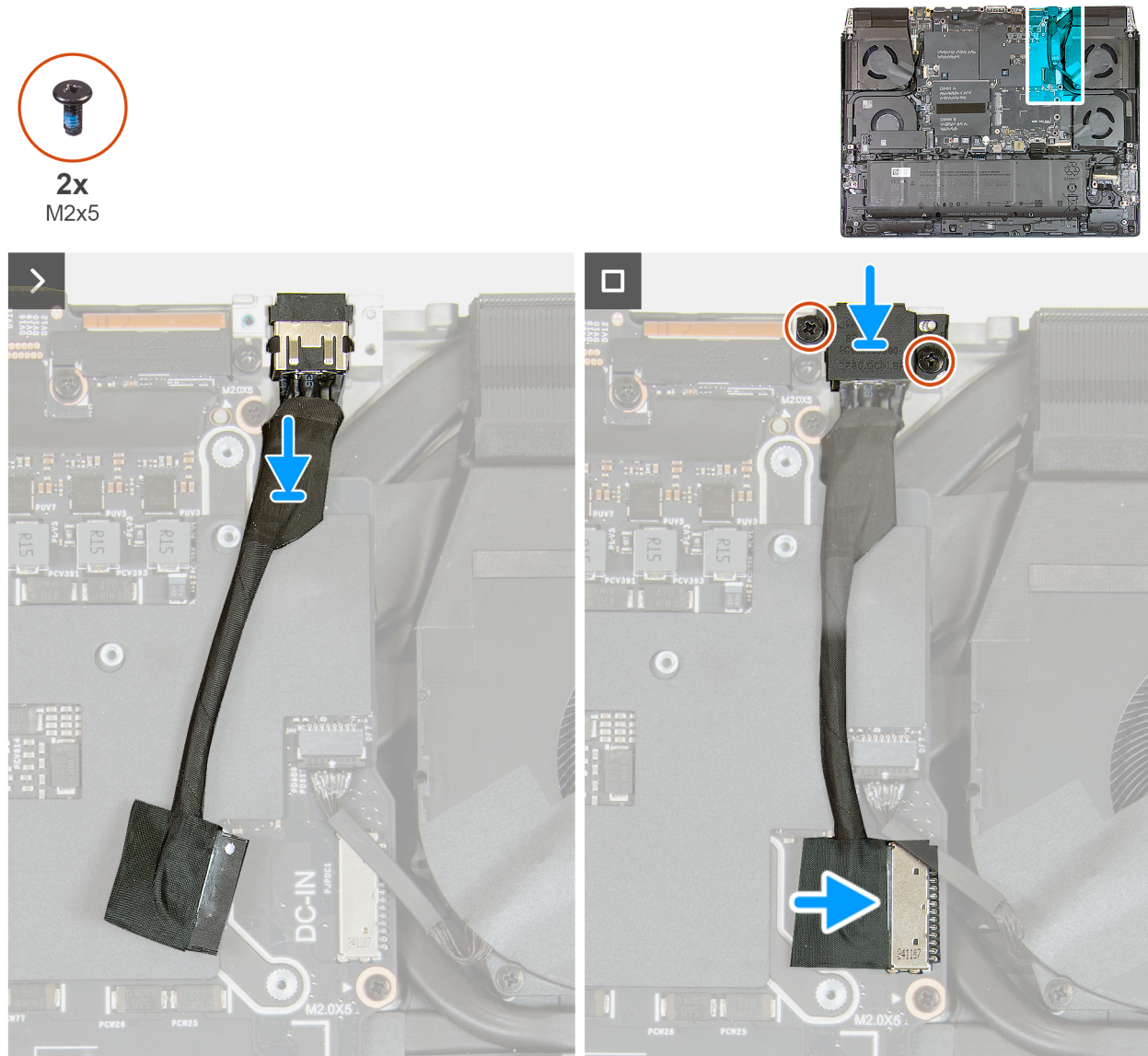
Abbildung 58. Einbauen des Netzadapteranschlusses
