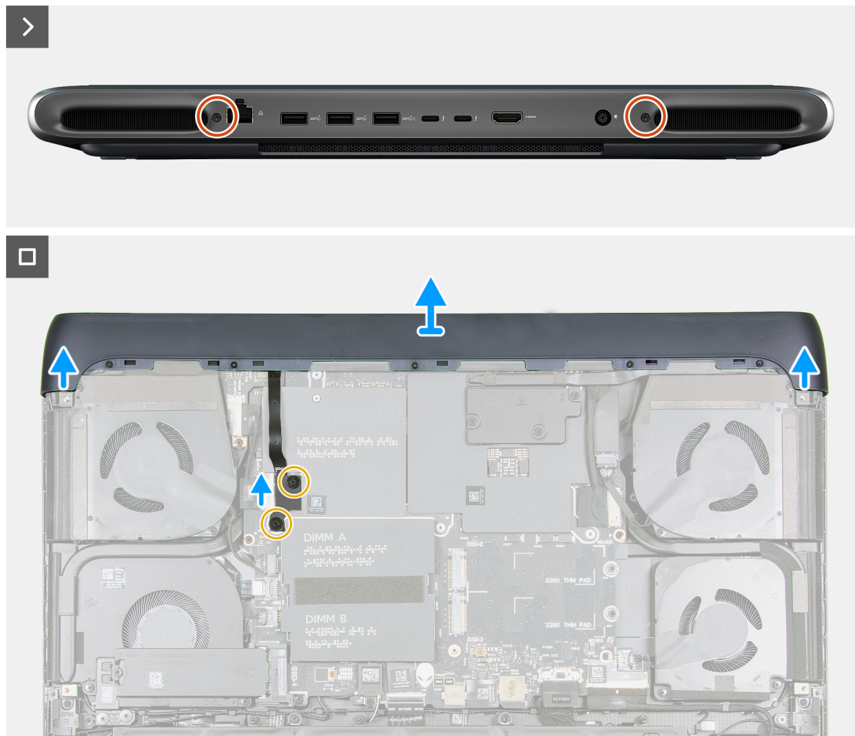
Abbildung 29. Entfernen der hinteren E/A-Abdeckung
