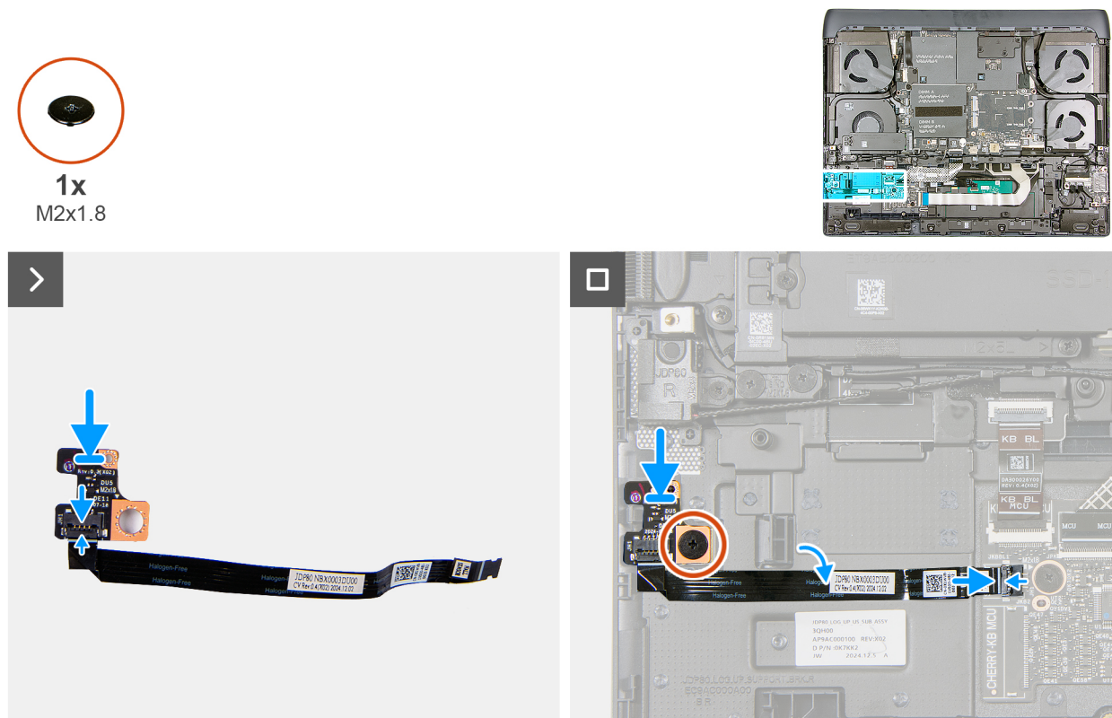
Abbildung 44. Installieren der Hall-Sensorplatine
