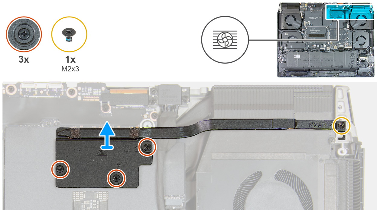
Abbildung 45. Entfernen des VR-Kühlkörpers
