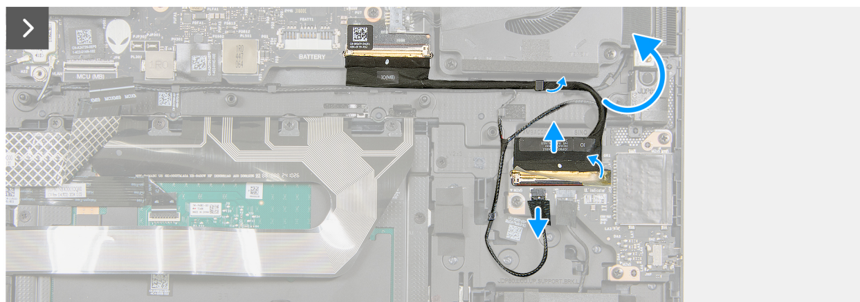
Abbildung 34. Entfernen der Hochtöner
