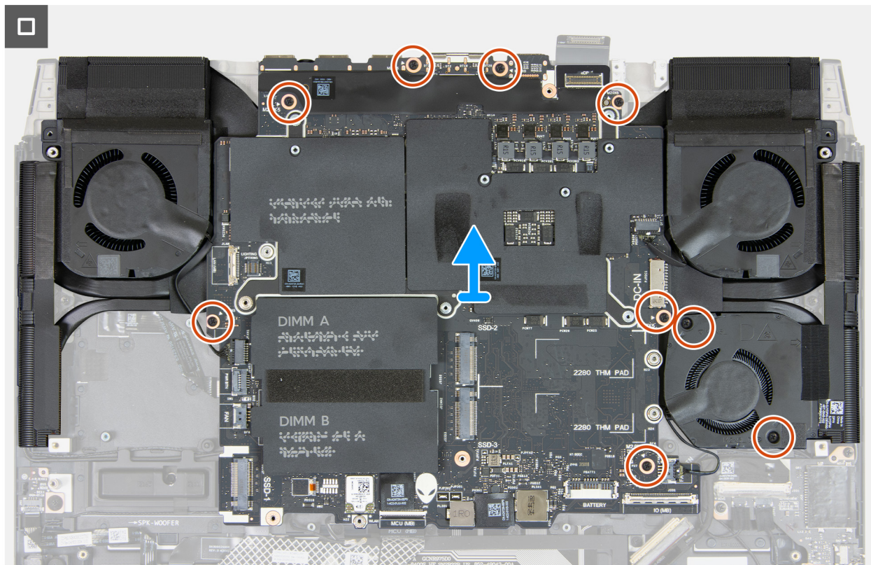
Abbildung 60. Entfernen der Systemplatine
