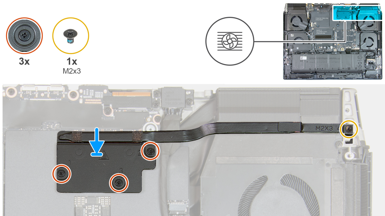
Abbildung 46. Installieren des VR-Kühlkörpers
