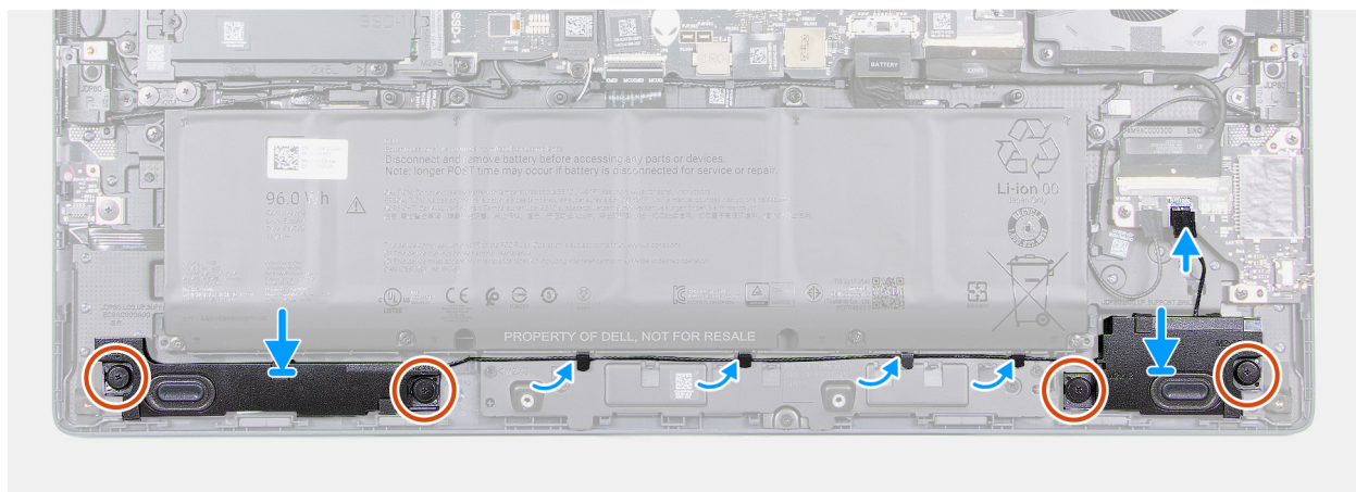
Abbildung 38. Einbauen der Woofer
