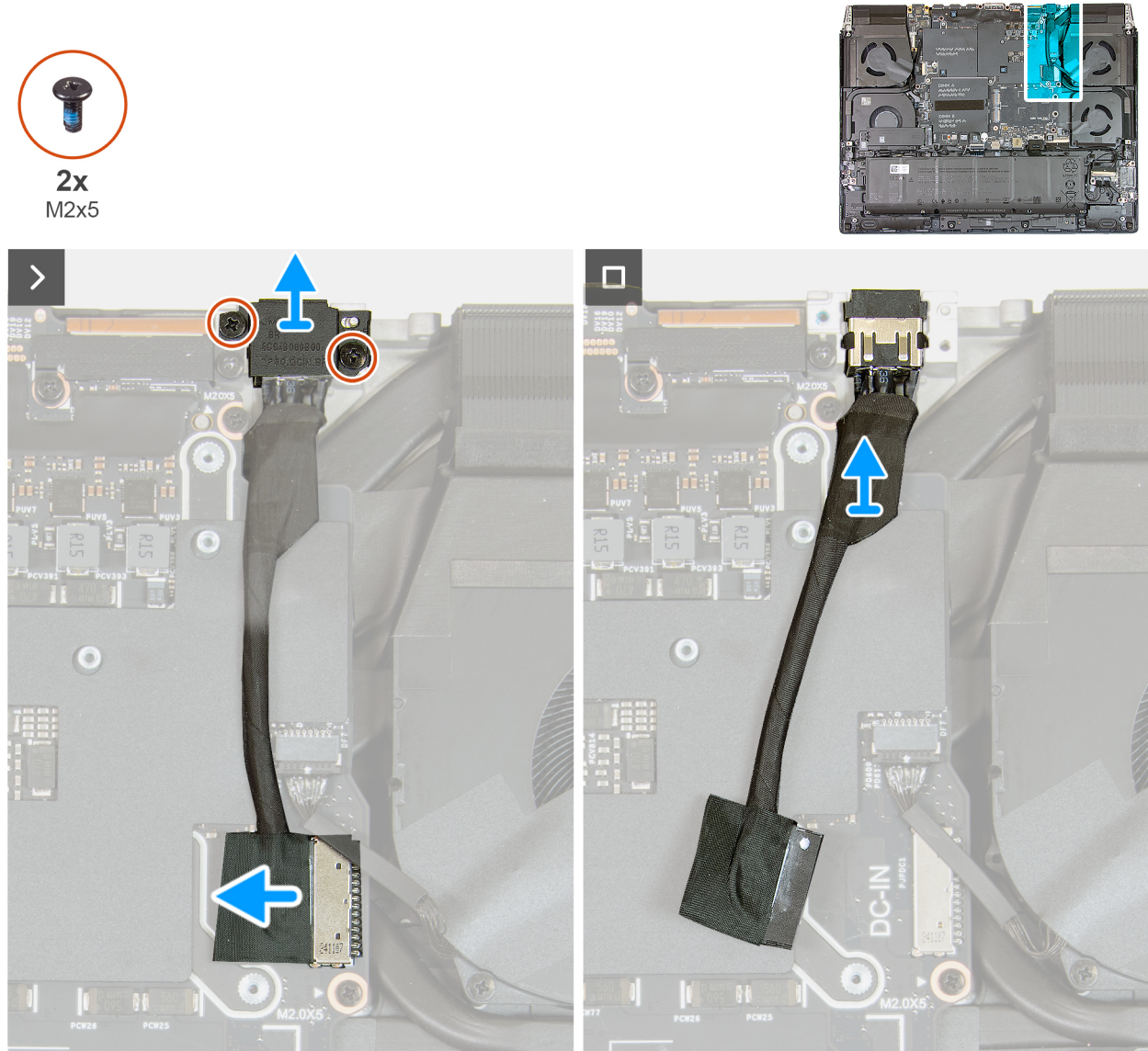
Abbildung 57. Entfernen des Netzadapteranschlusses
