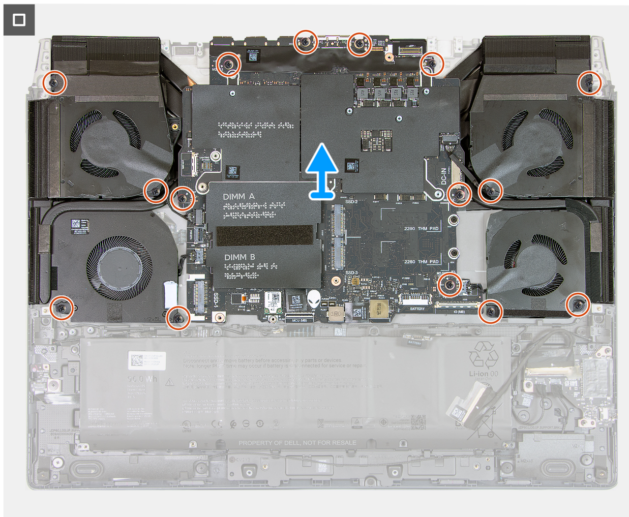
Abbildung 62. Trennen der Kabel von der Hauptplatine
