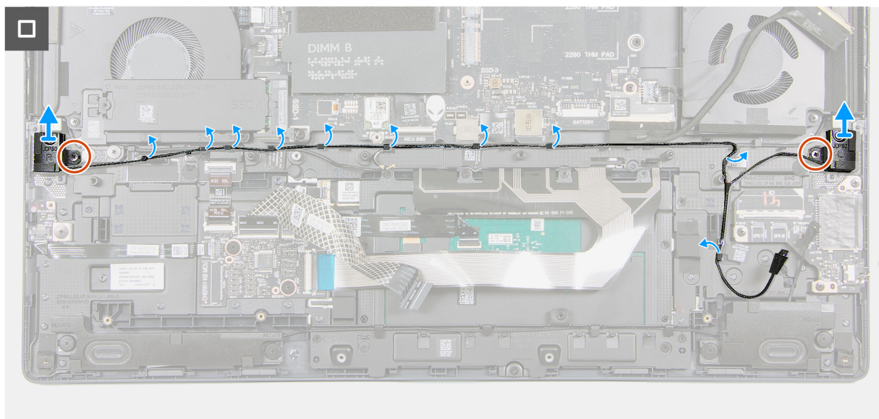
Abbildung 35. Entfernen der Hochtöner
