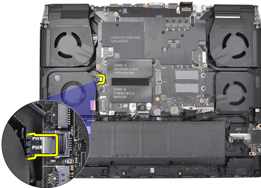
Abbildung 71. Anschluss für Netzschalter
