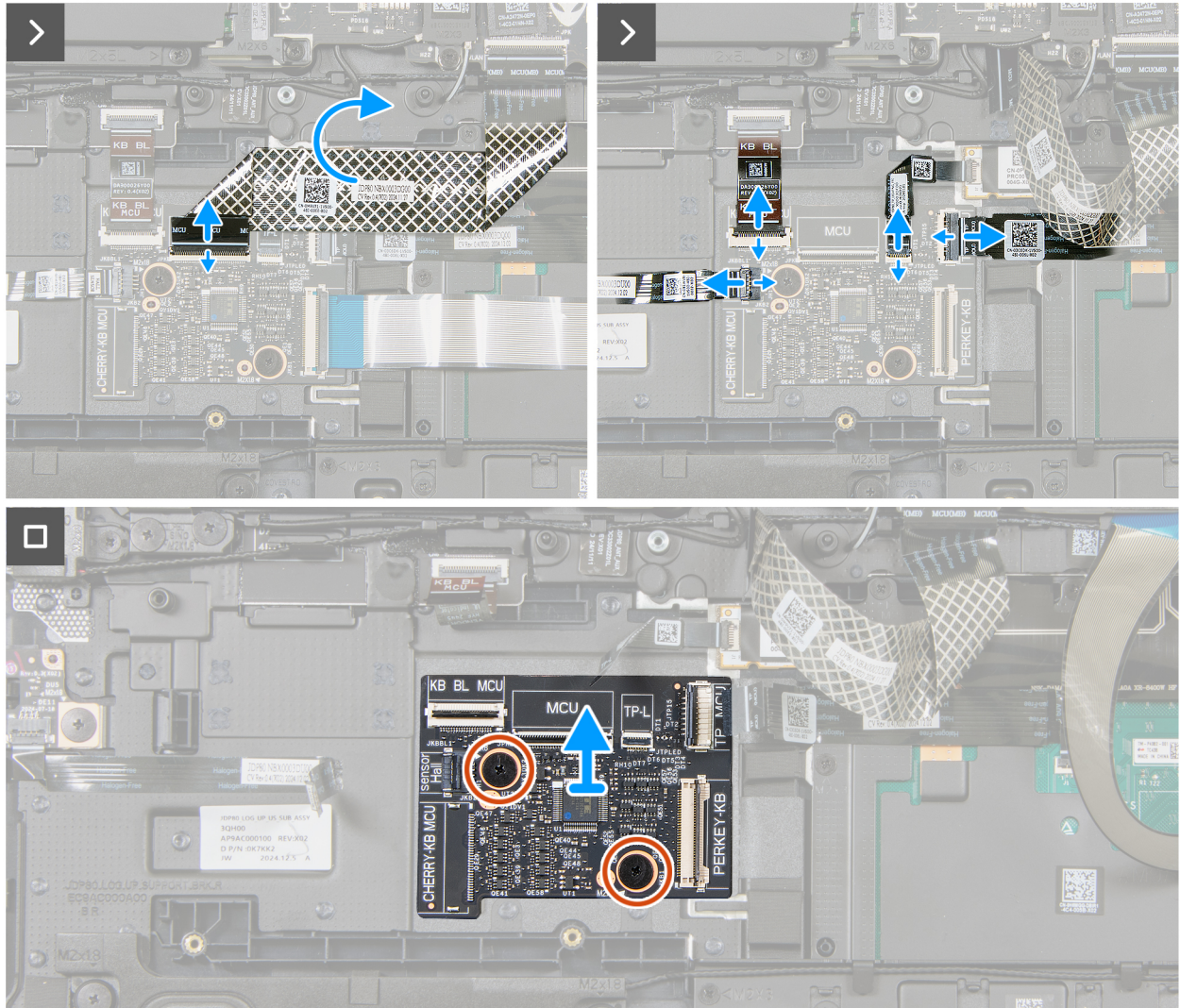
Abbildung 41. Entfernen der Tastatursteuerungsplatine
