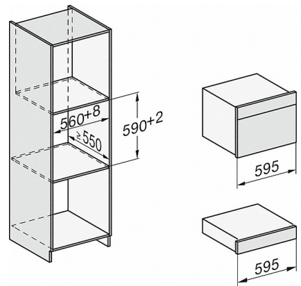
ESW7x10, Skizze
