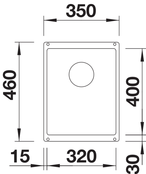
Aufsicht
