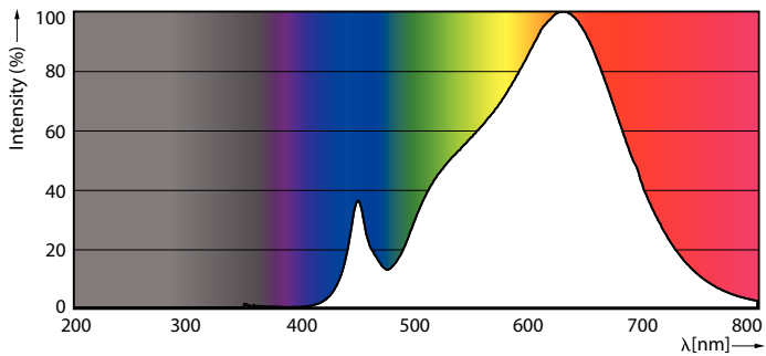
LEDbulb CLA 3,2W P45 E27 927 922 CL
