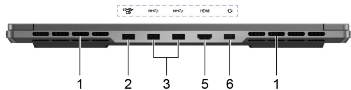
Abbildung 1. Rückansicht—Legion Slim 7 16IRH8 und Lenovo Legion Slim 7 16IRH8 D2
