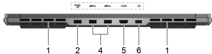
Abbildung 2. Rückansicht—Legion Slim 7 16APH8 und Lenovo Legion Slim 7 16APH8 D2
