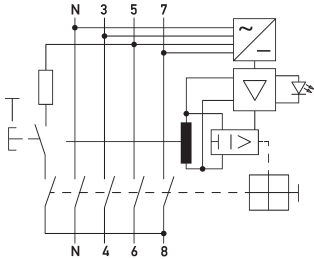
Anschlusschema
