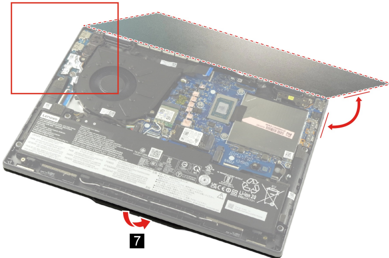
Figure 26. Remove the display module
