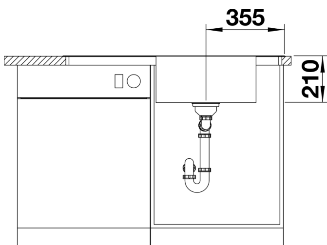
Frontansicht
