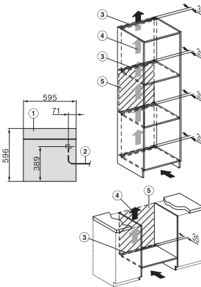
DGC7x60 Anschlüsse und Belüftung 60cm, Skizze
