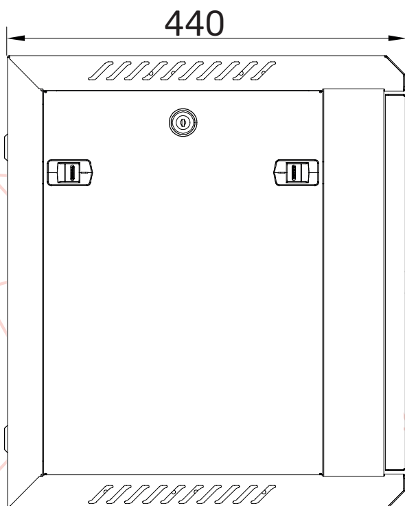
Seitenansicht
