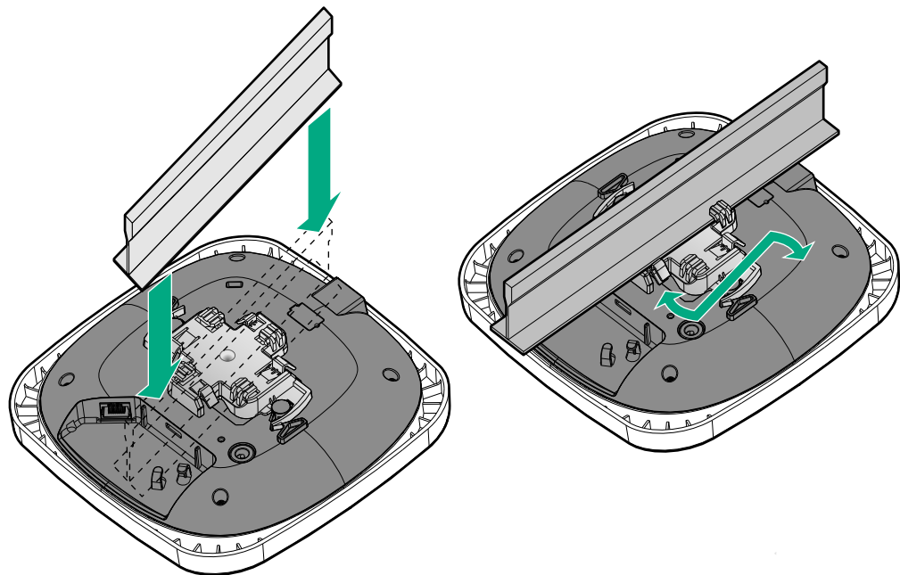
Abbildung 7 Montieren des AP an einer 9/16-Zoll-Deckenschiene
