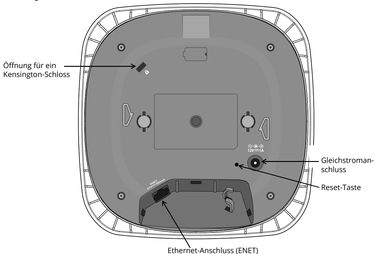
Abbildung 2 Rückseite
