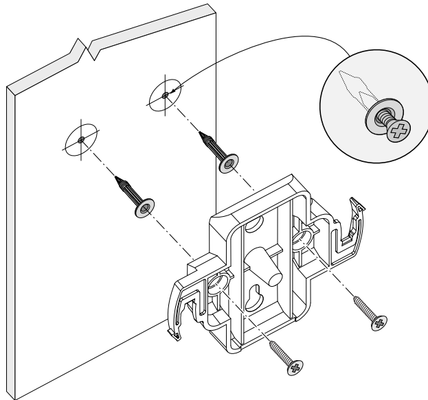
Abbildung 9 Befestigen der Montageklammer an einer massiven Fläche
