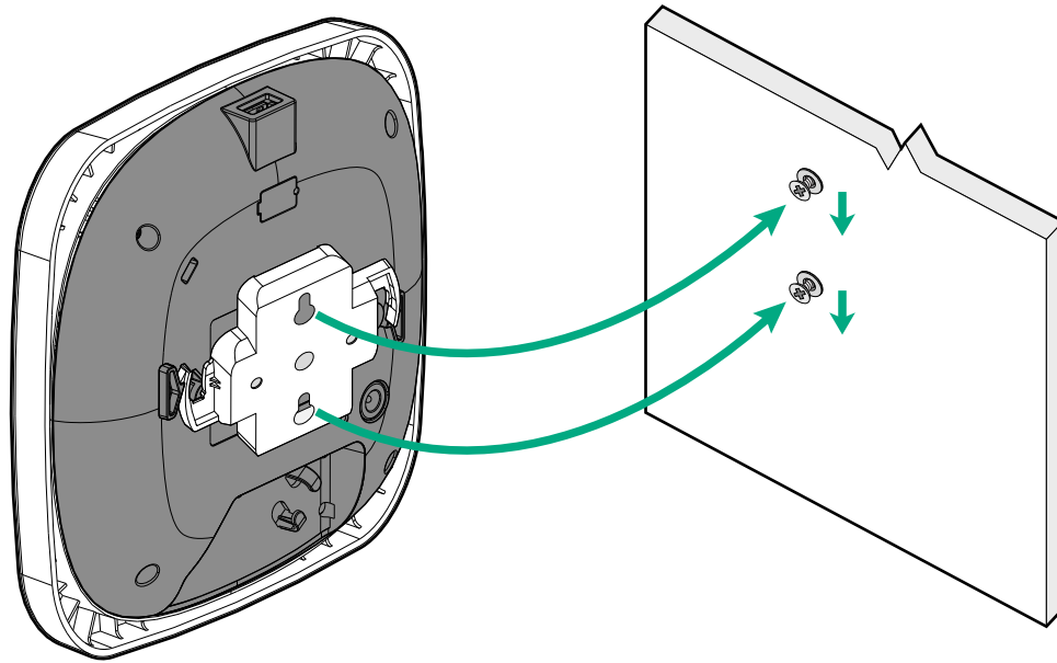
Abbildung 12 Montage der Halterung mit AP an der Wand
