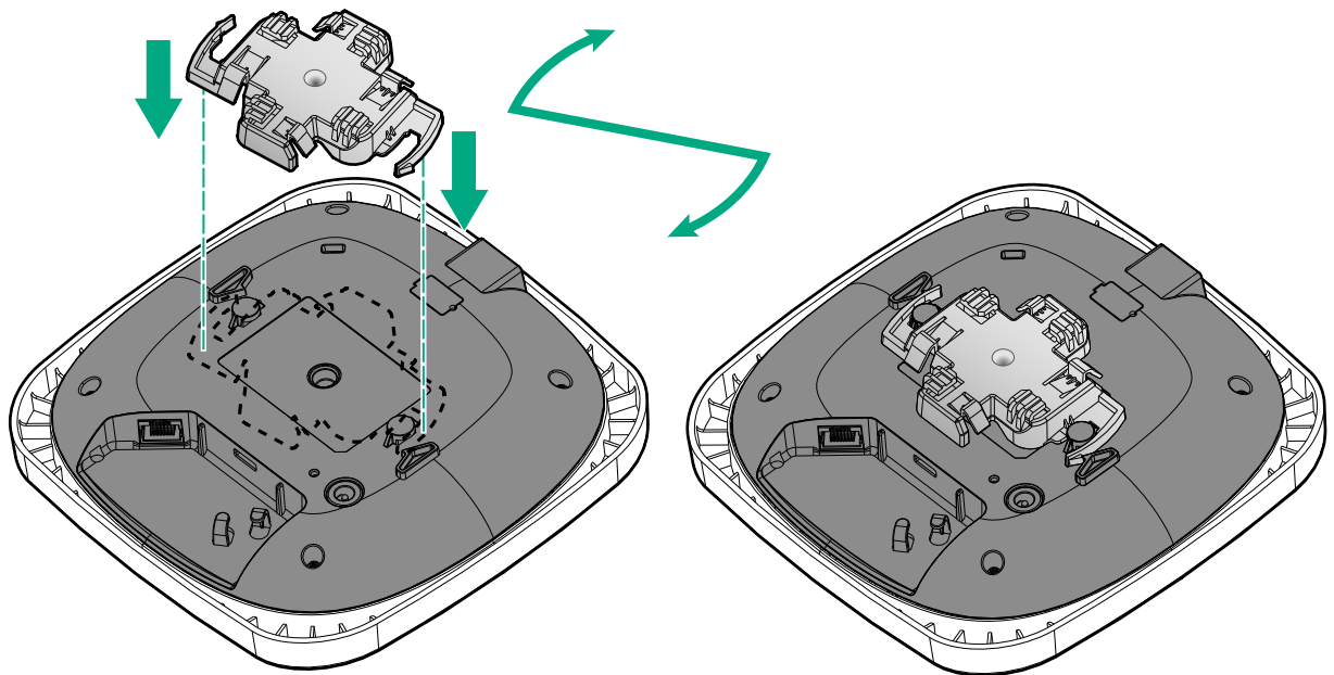
Abbildung 5 Anbringen des Deckenschienenadapters am AP
