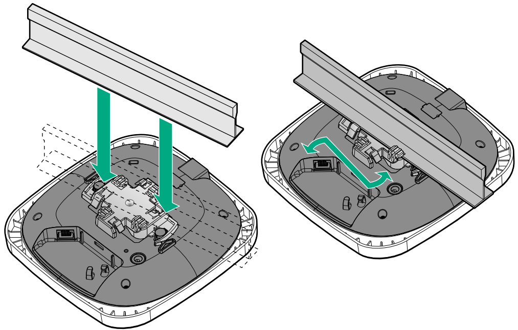
Abbildung 6 Montieren des AP an einer 15/16-Zoll-Deckenschiene
