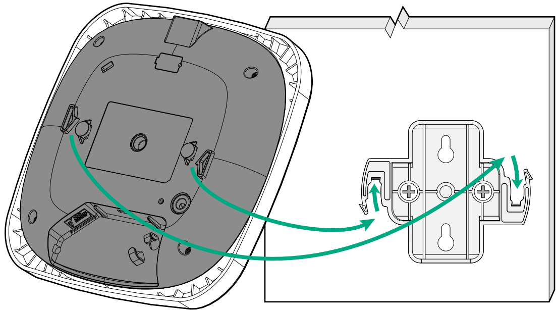
Abbildung 10 Befestigen des AP an der Montagehalterung
