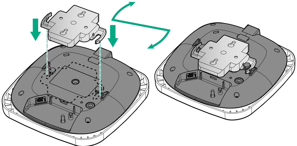
Abbildung 11 Montage der Halterung
