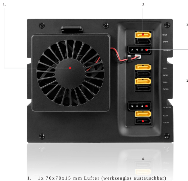
Rückansicht IB-544SSK
