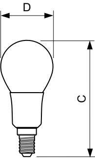
filament 2.5W-25W 250lm NAD 2700K E14D
